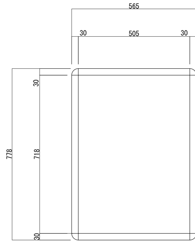
【正面図 S=1:10】
