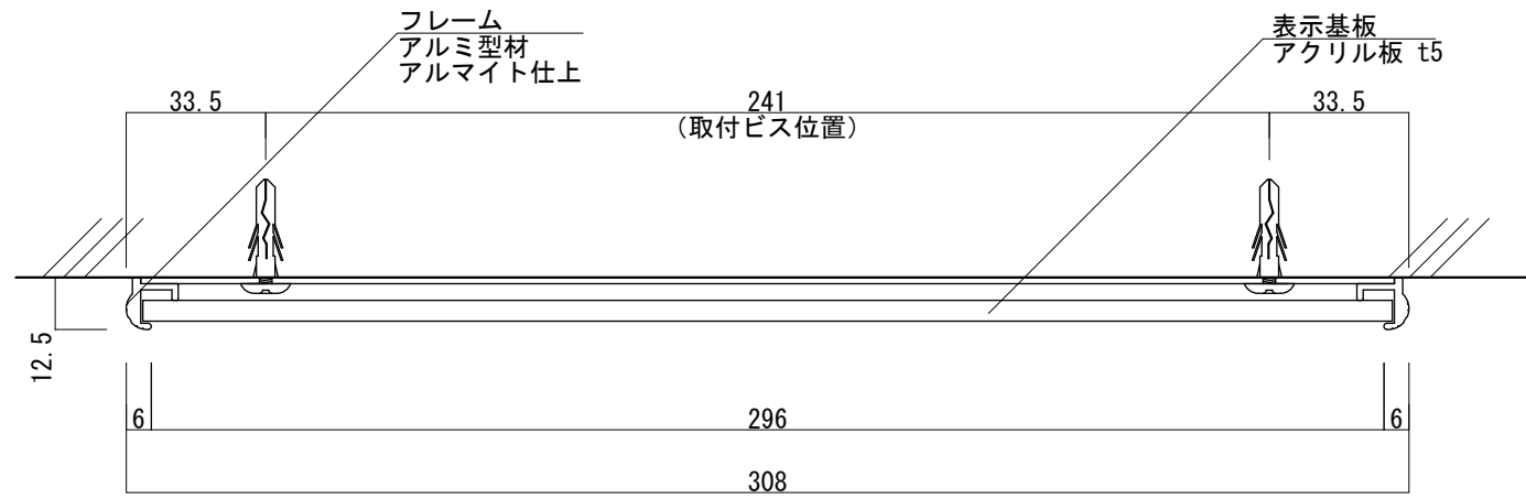
【平面図 S=1:2】
