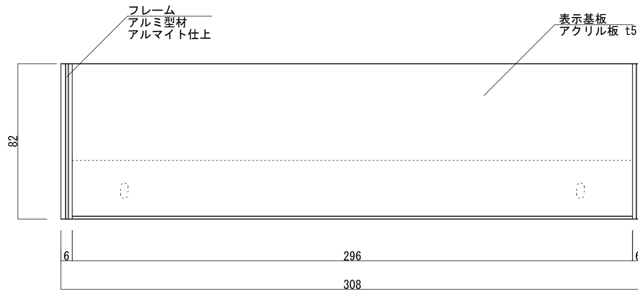
【正面図 S=1:2】
