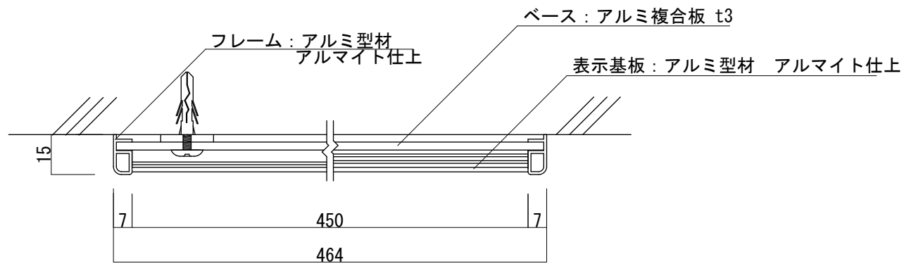
【平面図 S=1:2】
