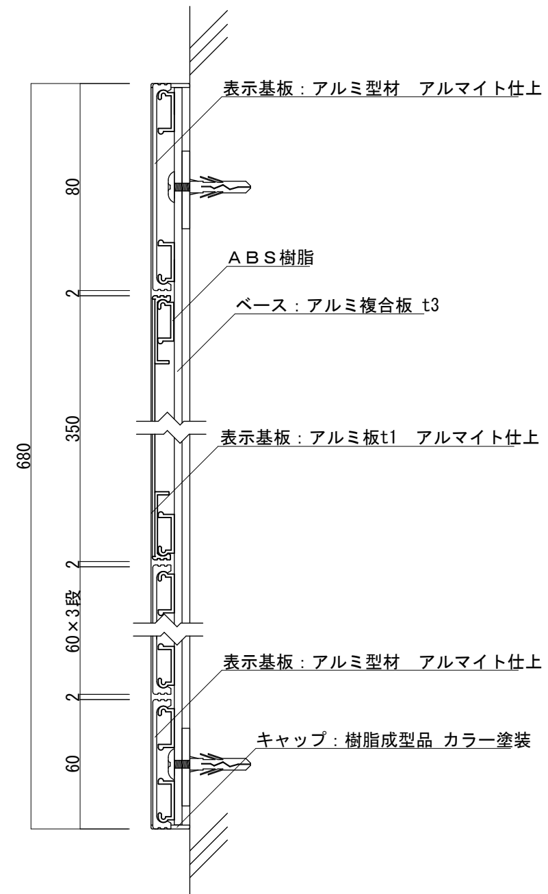
【側面図 S=1:2】
