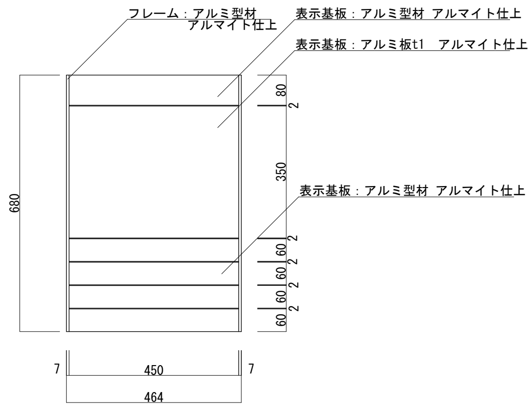
【正面図 S=1:10】
