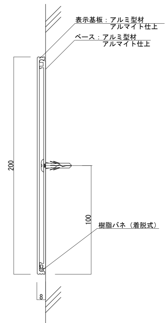
【側面図 S=1:2】
