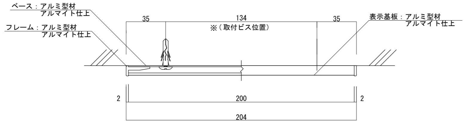
【平面図 S=1:2】
