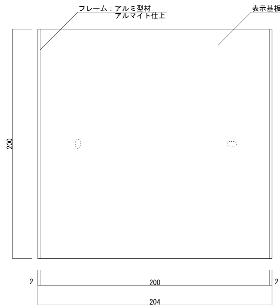
【正面図 S=1:2】
