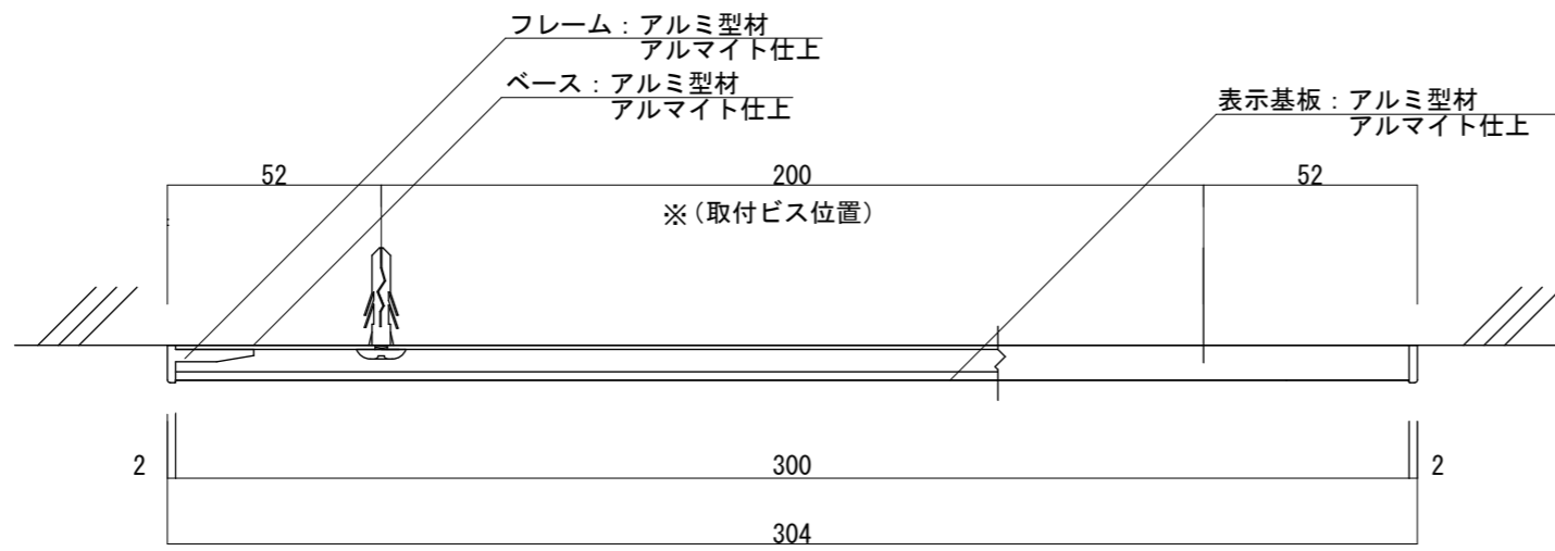
【平面図 S=1:2】
