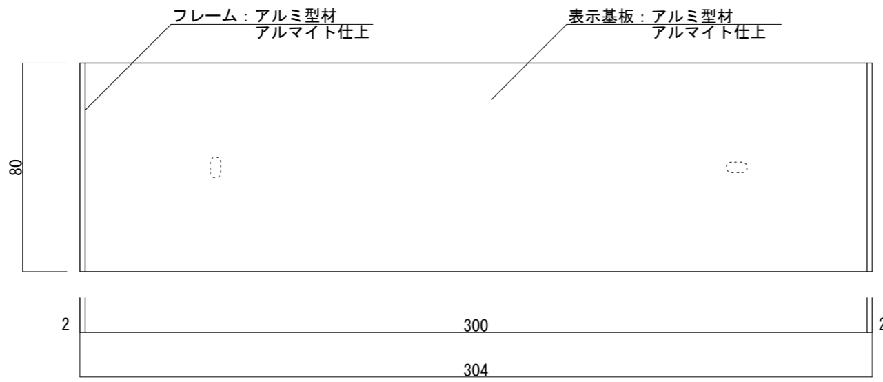
【正面図 S=1:2】
