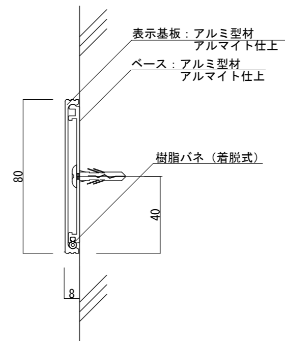
【側面図 S=1:2】
