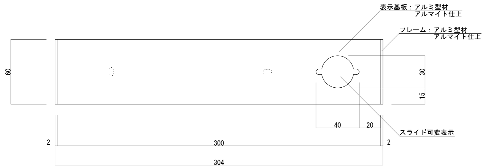
【正面図 S=1:2】
