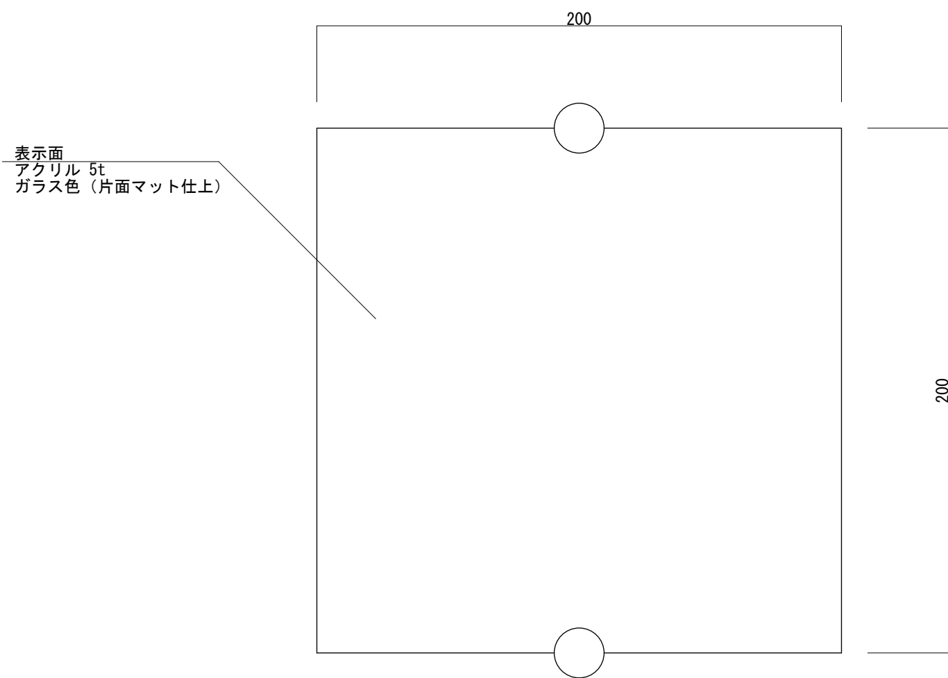
【正面図 S=1:2】
