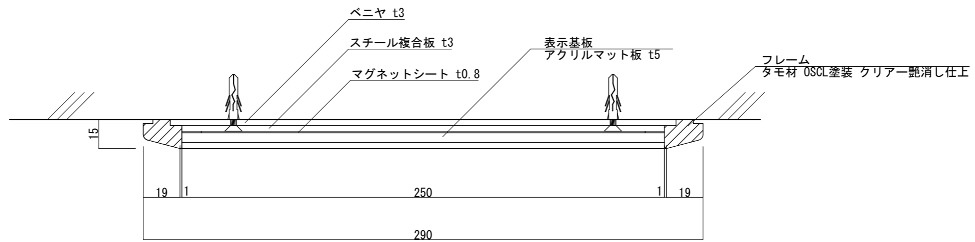
【平面図 S=1:2】
