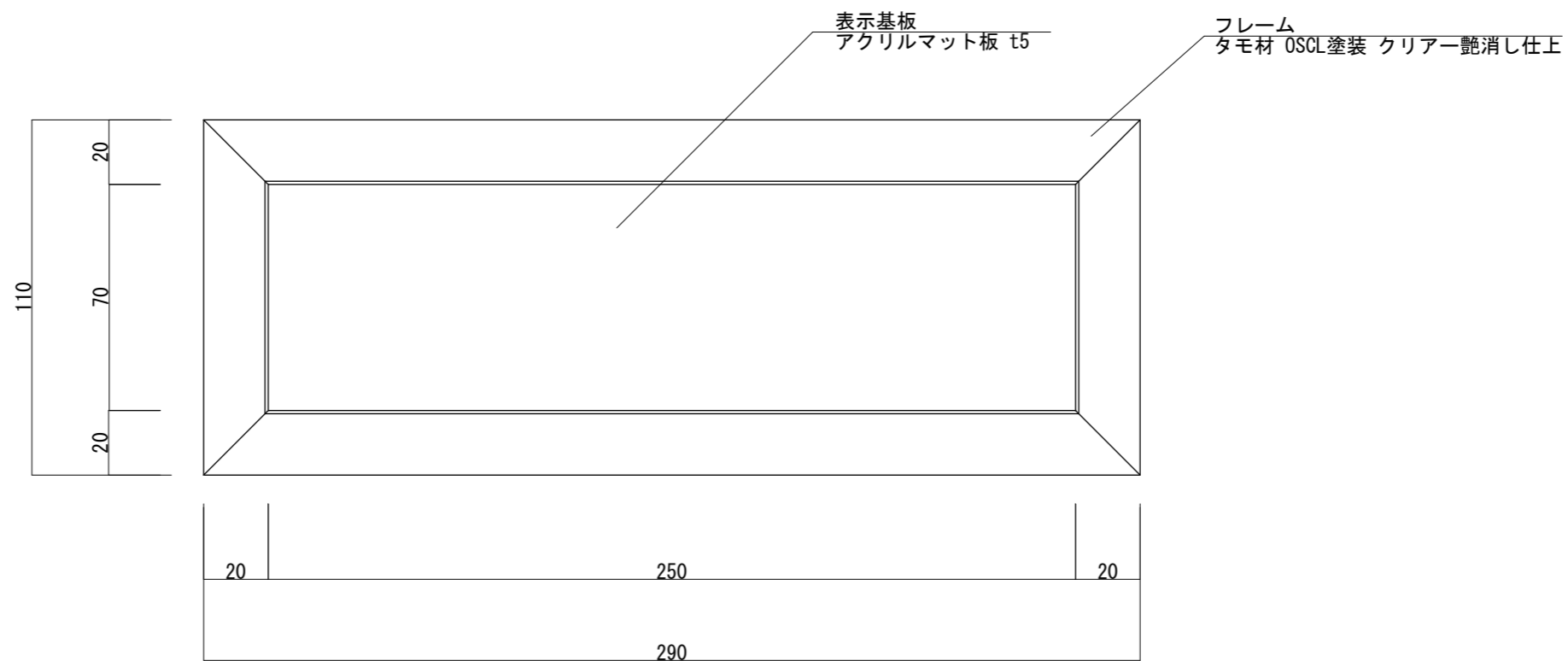
【正面図 S=1:2】
