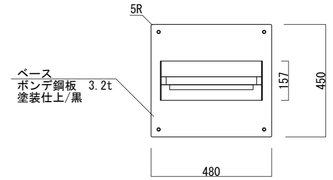
【平面図 S=1:15】
