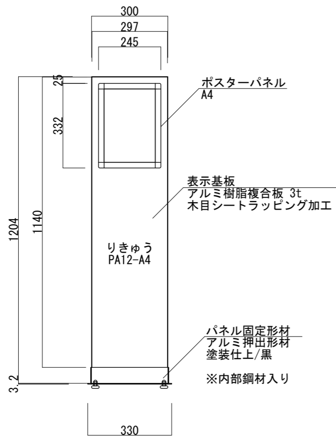
【正面図 S=1:15】
