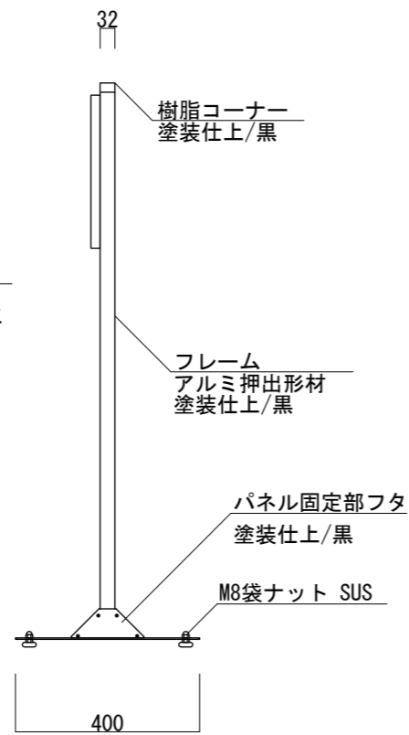
【側面図 S=1:15】
