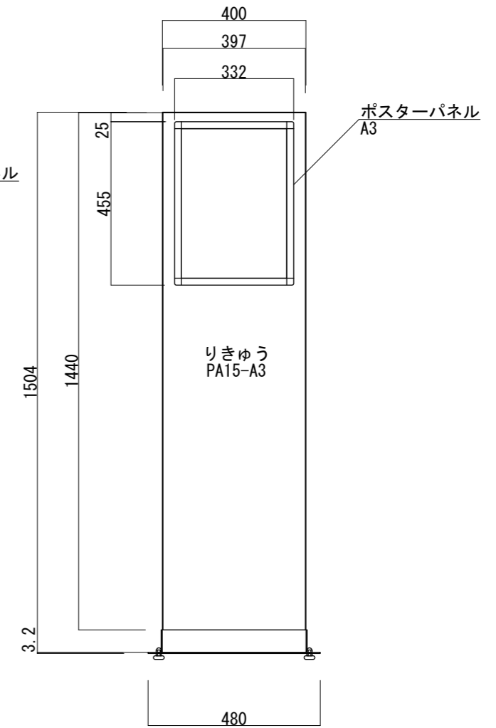
【正面図 S=1:15】
