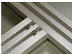
大型フレームには複数使用で剛性を確保
