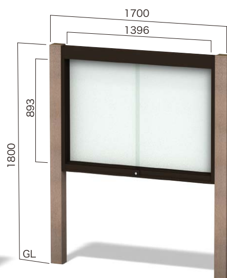
RGP-1510 照明なし ガラス引違いタイプ 設計価格 ¥300,000(外税) 埋込寸法 500mm 本体重量 53kg リサイクルエコウッド支柱
