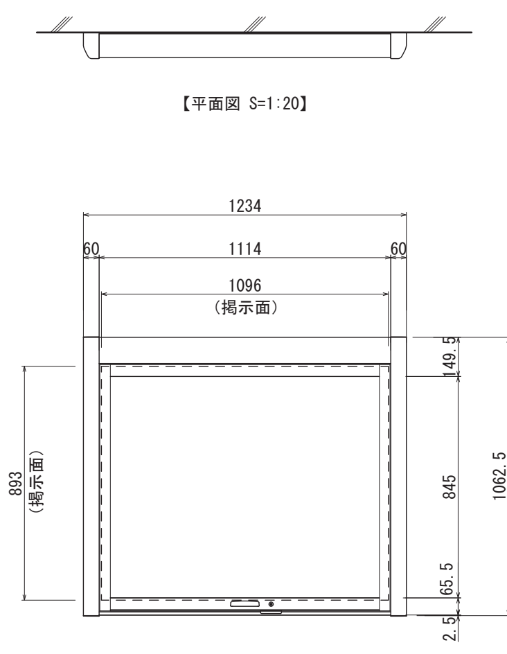
【正面図 S=1:20】
