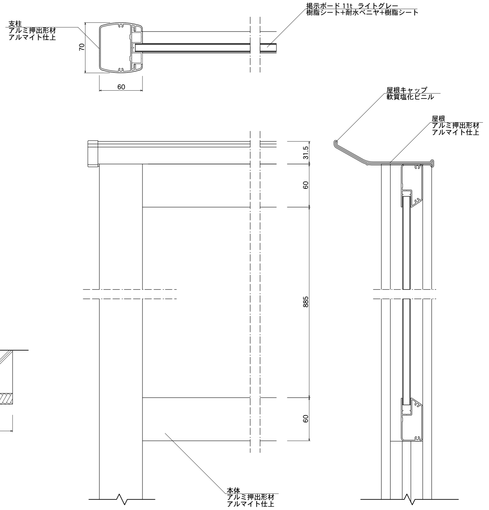
【側面図】
