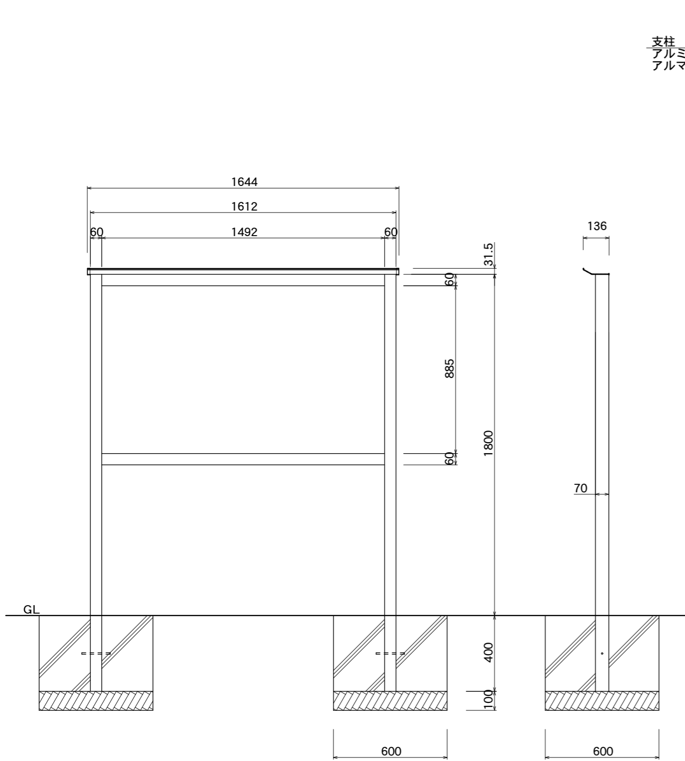
【正面図】
