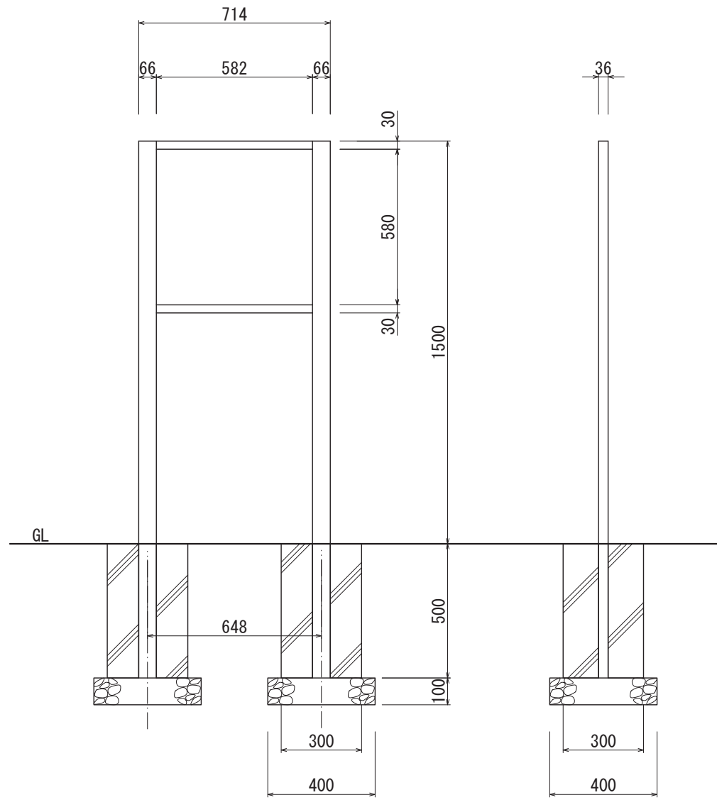
【正面図 S=1:20】
