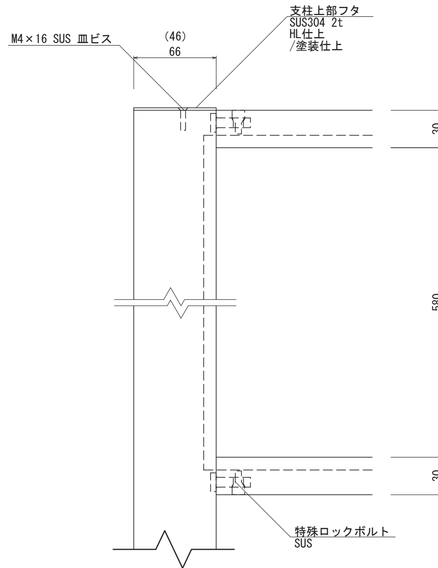
【正面図 S=1:3】
