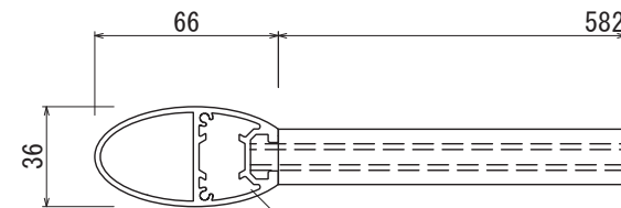
【平面図 S=1:3】
