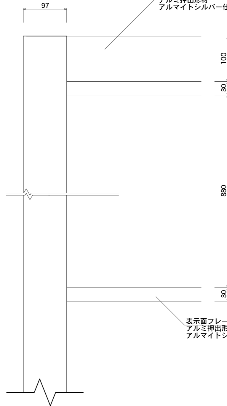
【正面図】
