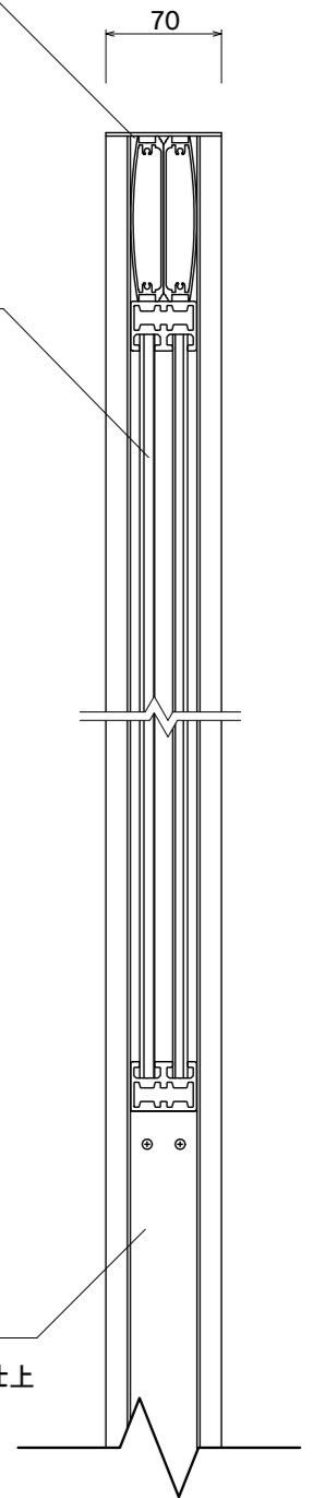
【側断面図】
