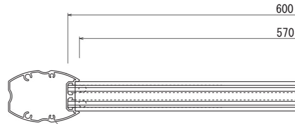
【平面図 S=1:5】
