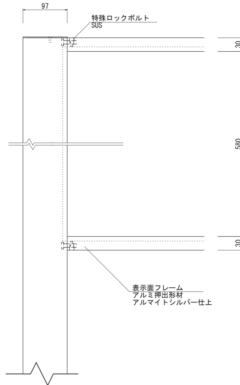
【正面図 S=1:5】
