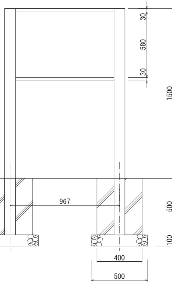
【正面図 S=1:20】
