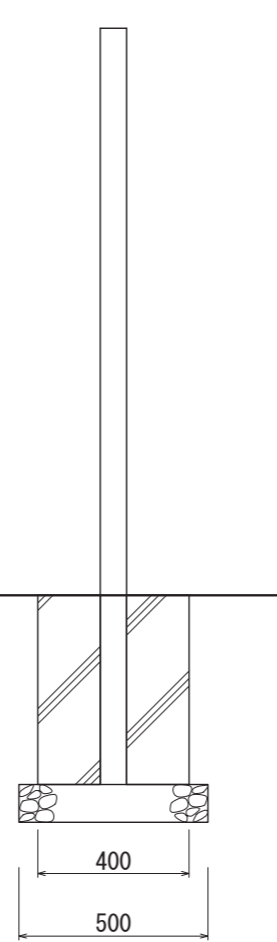
【側面図 S=1:20】
