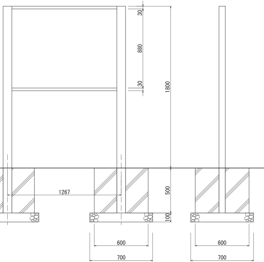
【正面図 S=1:20】
