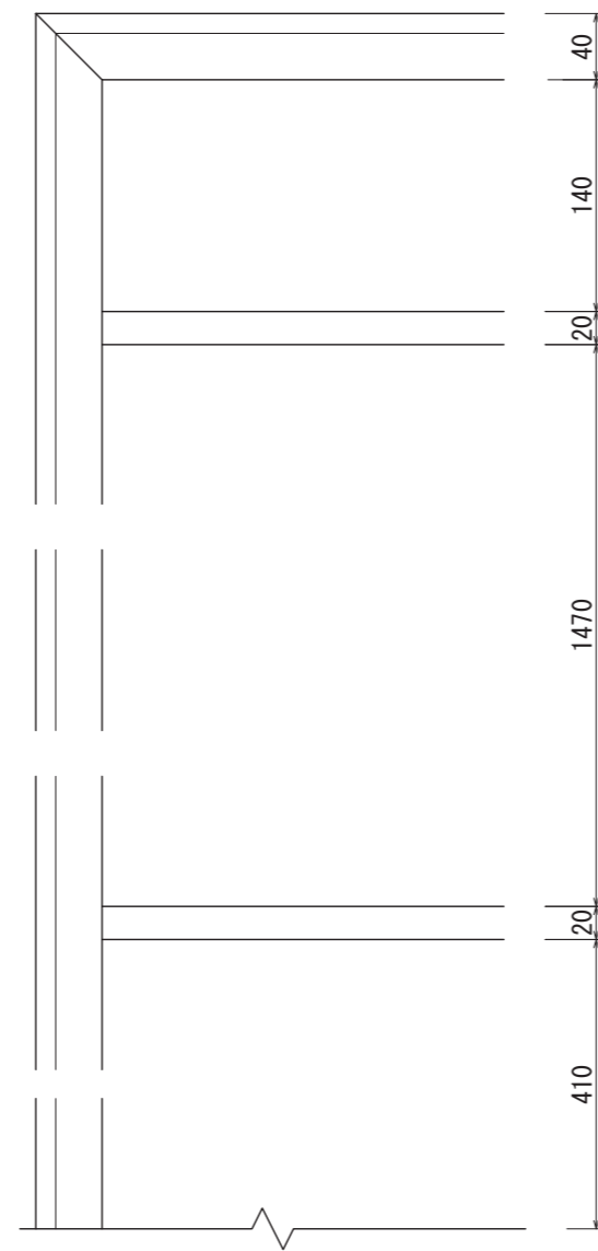
【正面図 S=1:5】
