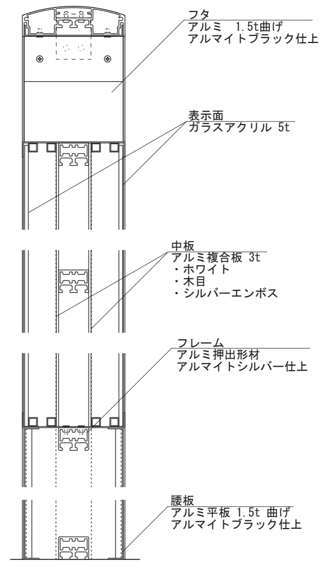
【側面図 S=1:5】
