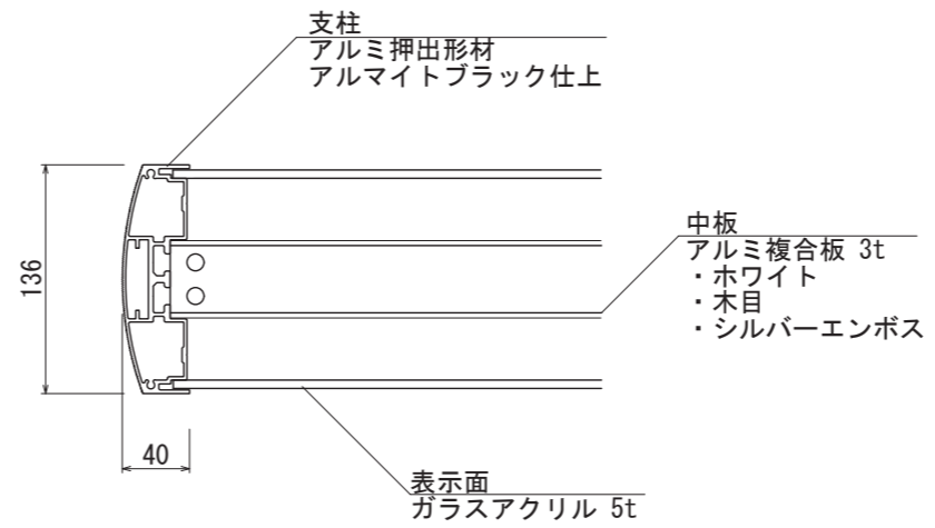
【平面図 S=1:5】
