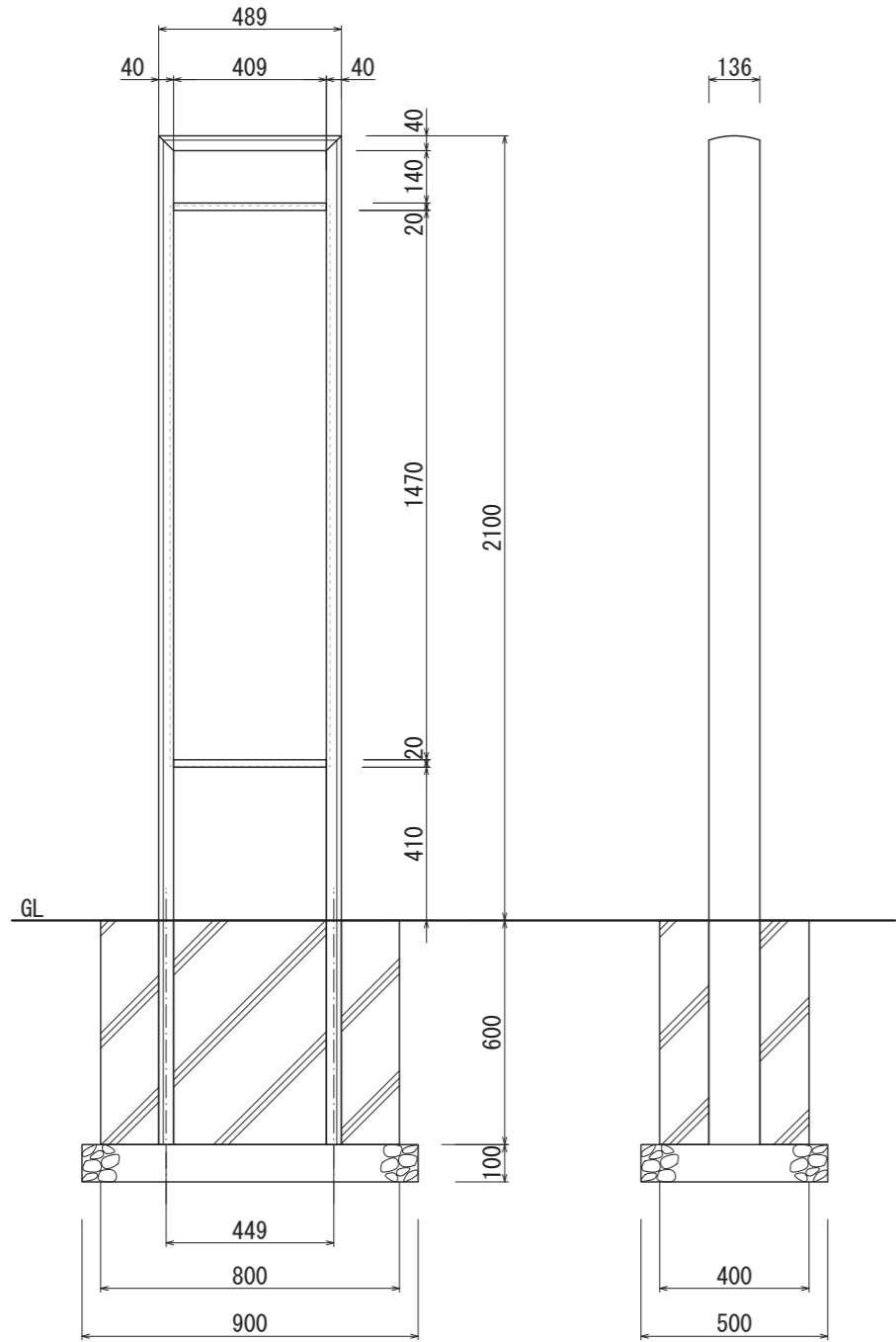
【正面図 S=1:20】
