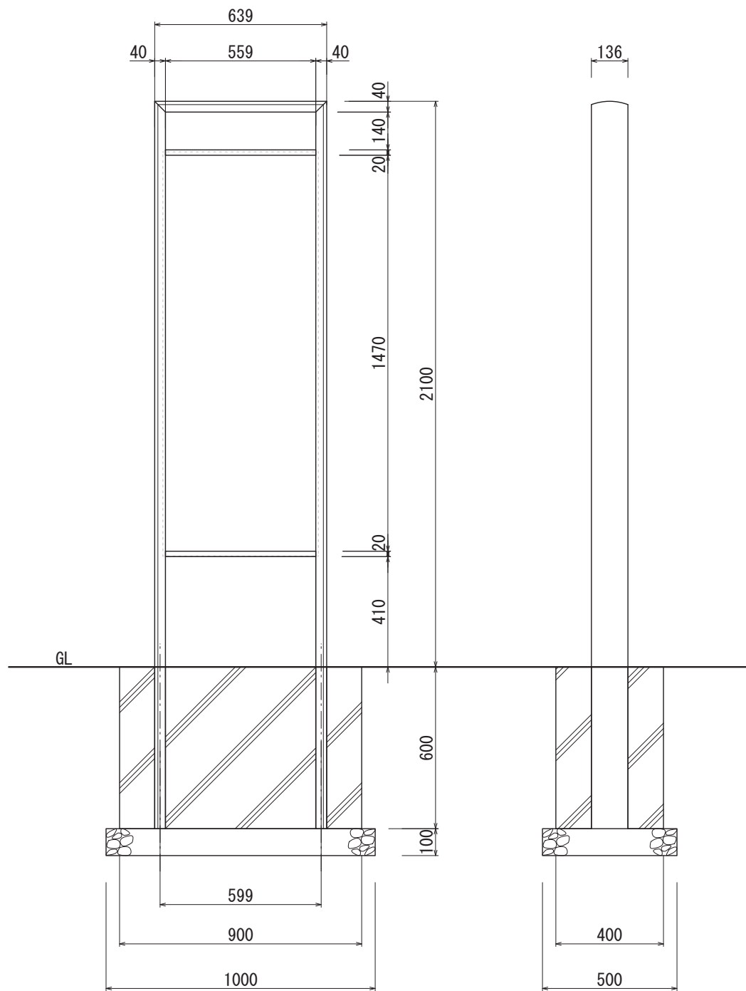
【正面図 S=1:20】
