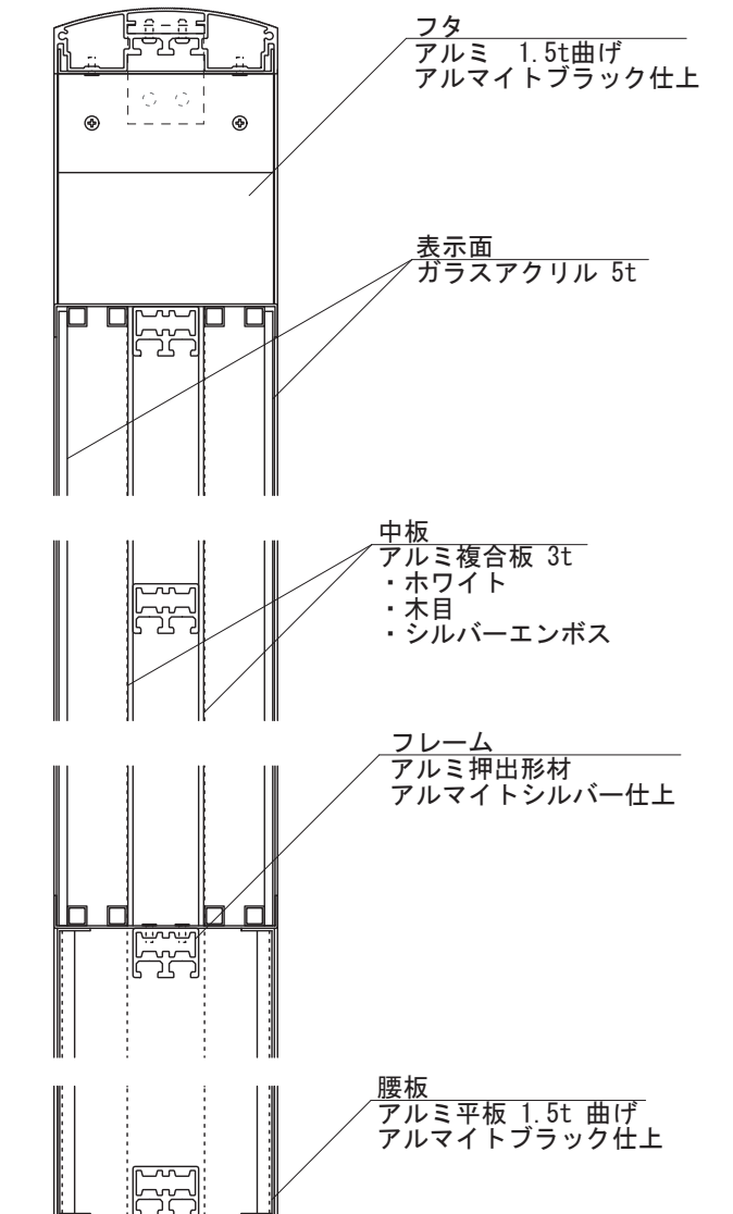
【側面図 S=1:5】
