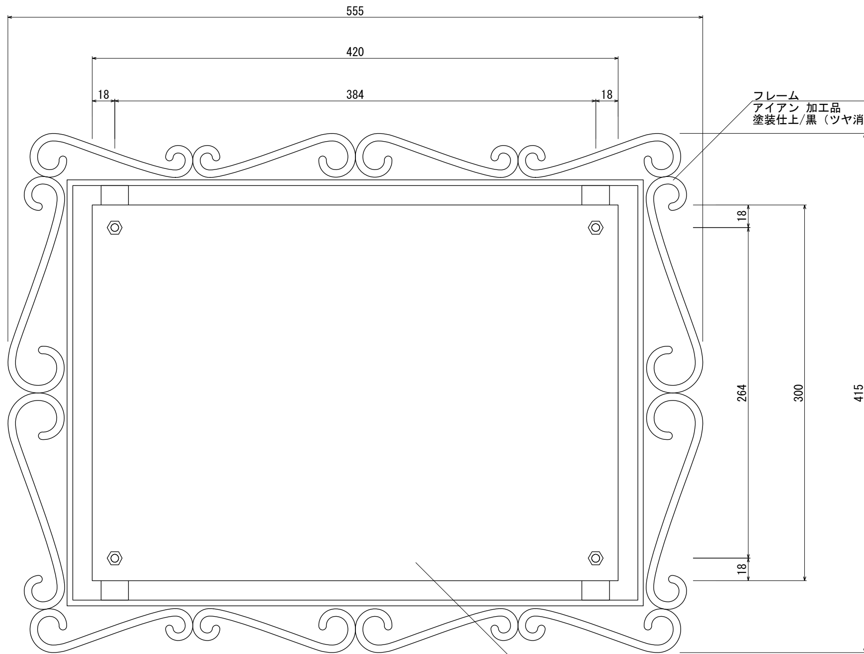
【正面図 S=1:3】
