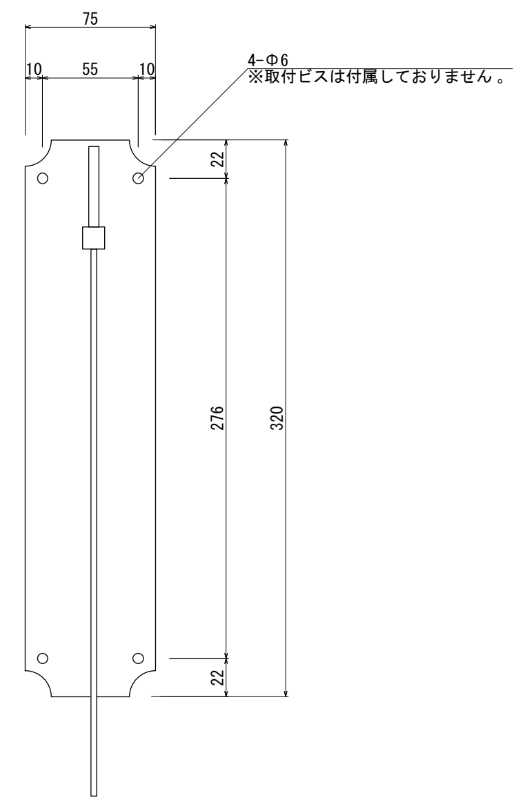
【側面図 S=1:3】
