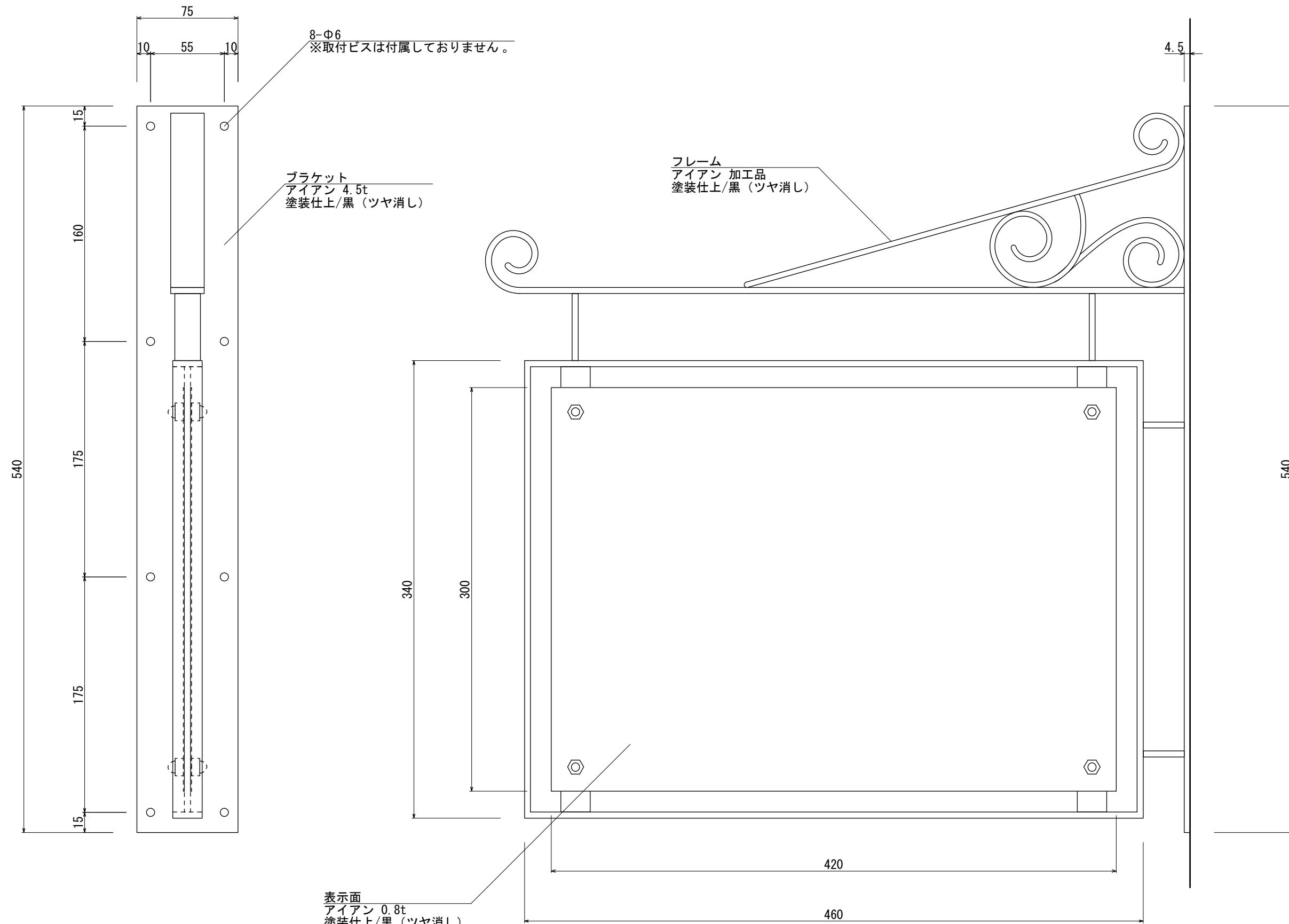
【側面図 S=1:3】
