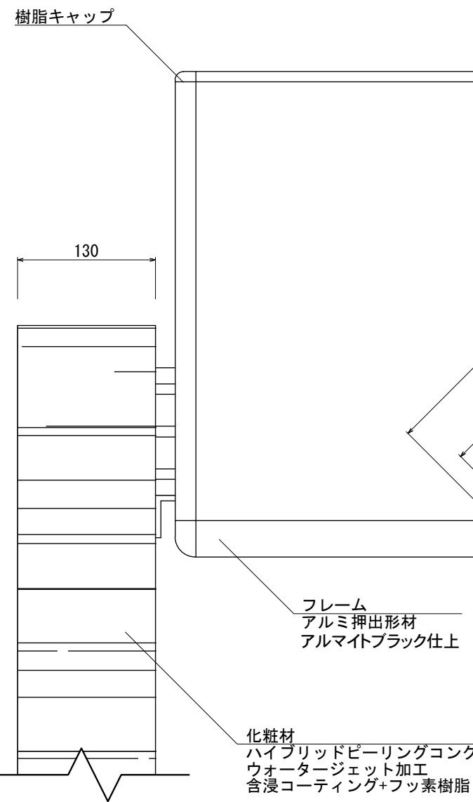
【正面図 S=1:5】
