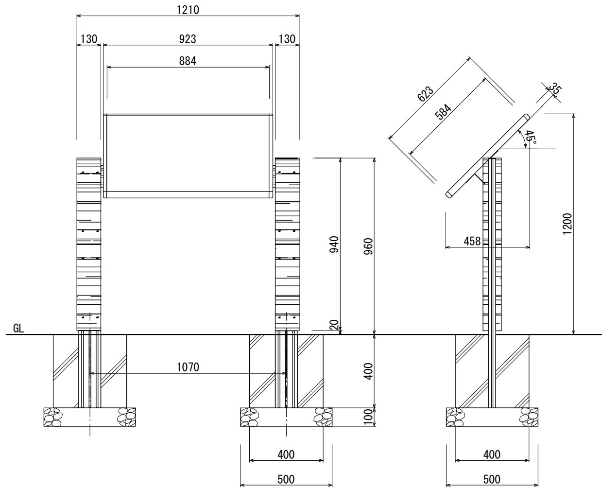
【正面図 S=1:20】
