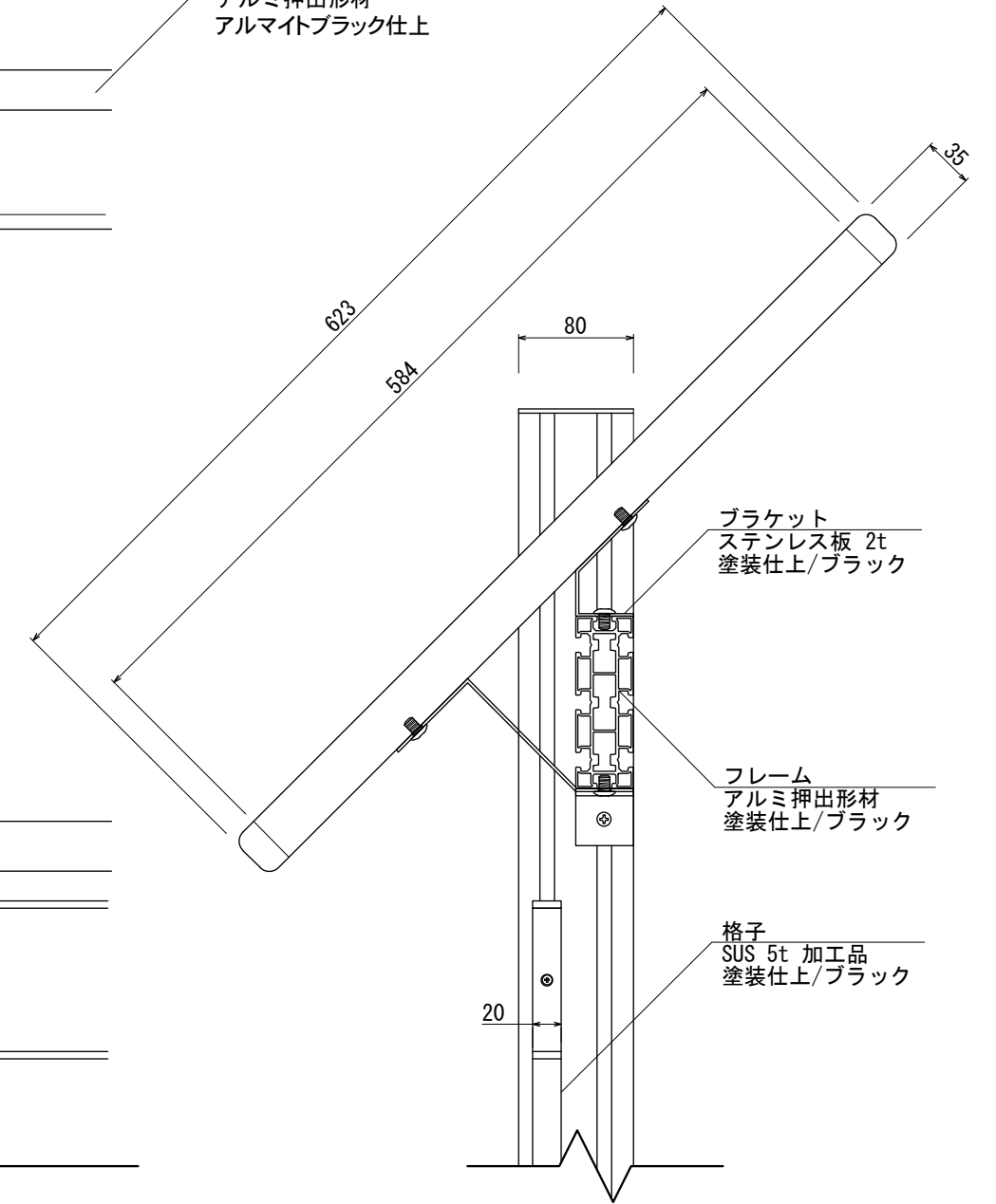
【正面図 S=1:5】
