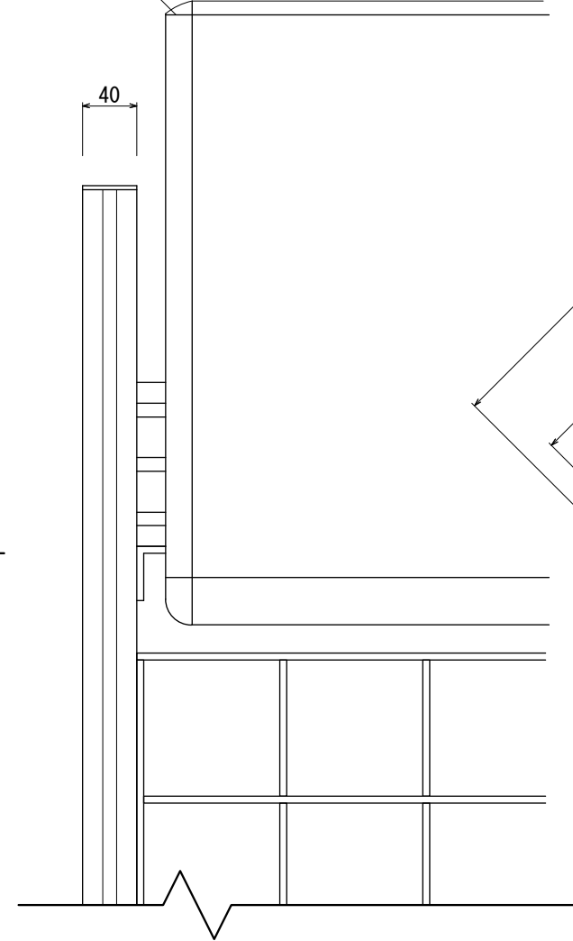
【正面図 S=1:5】
