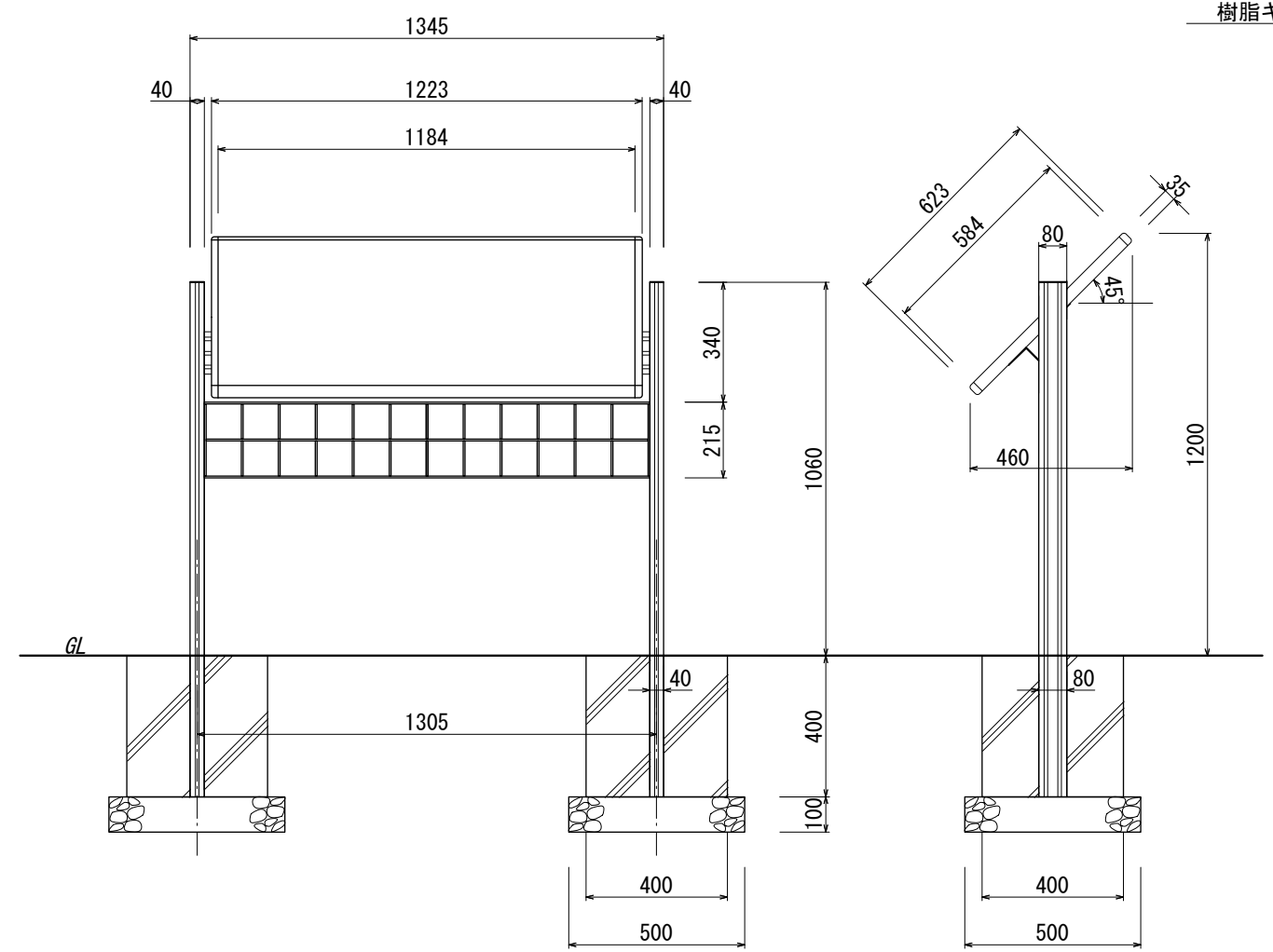
【正面図 S=1:20】
