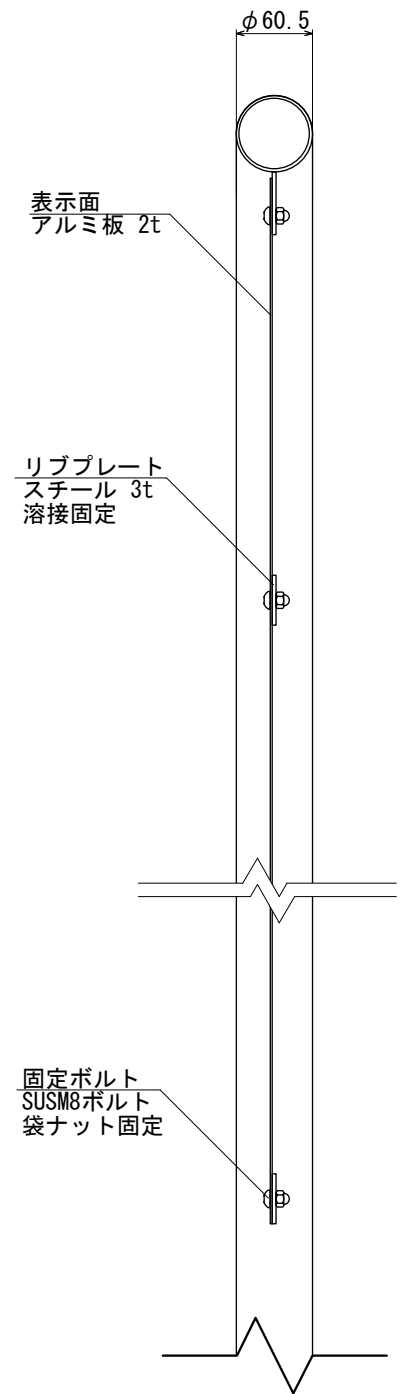
【側断面図 S=1:6】
