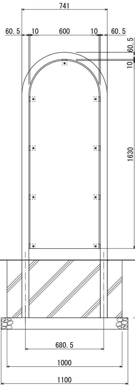
【正面図 S=1:20】
