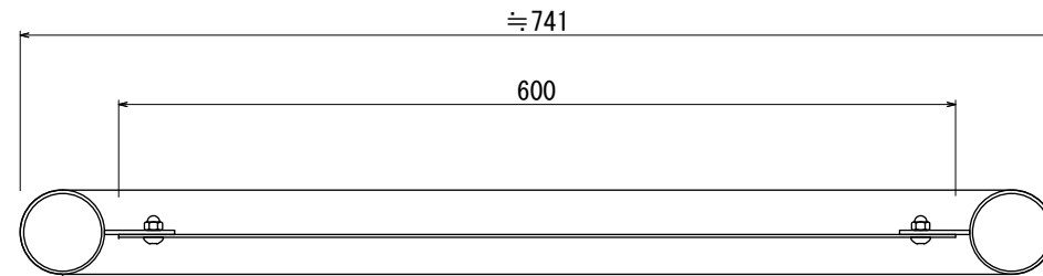
【平面図 S=1:6】
