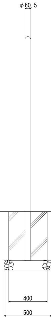
【側面図 S=1:20】
