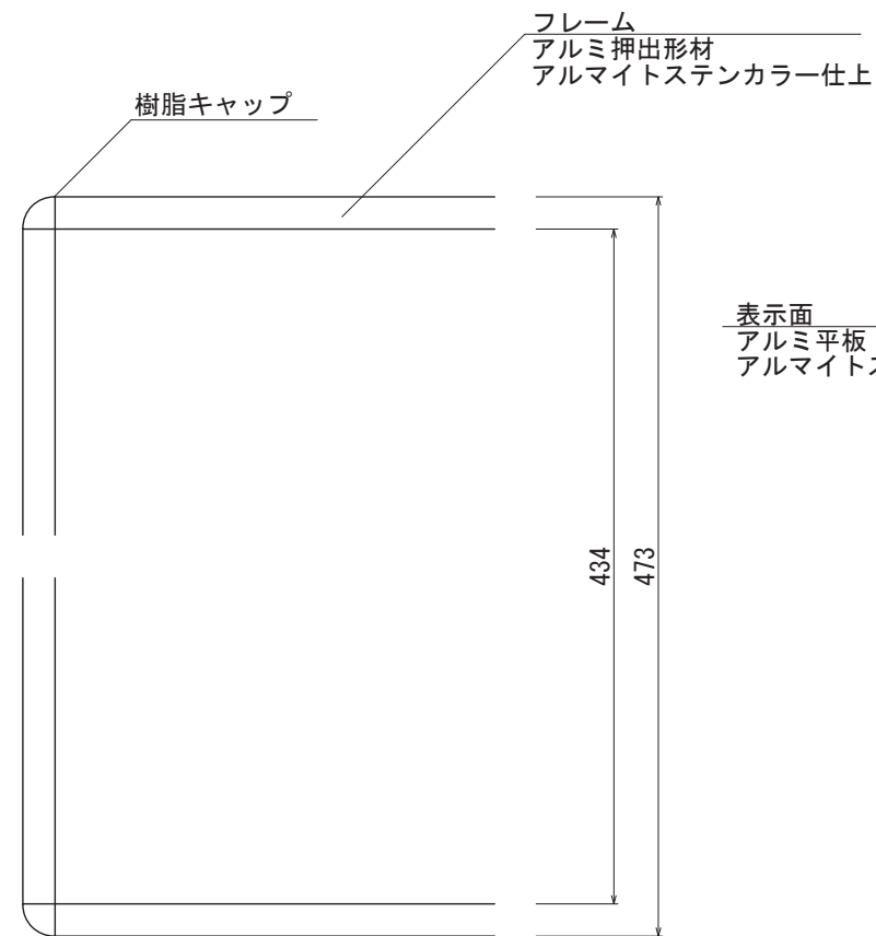
【平面図 S=1:5】
