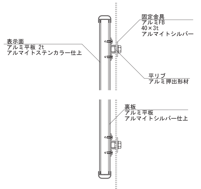
【側面図 S=1:5】
