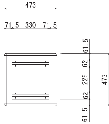
【背面図 S=1:20】
