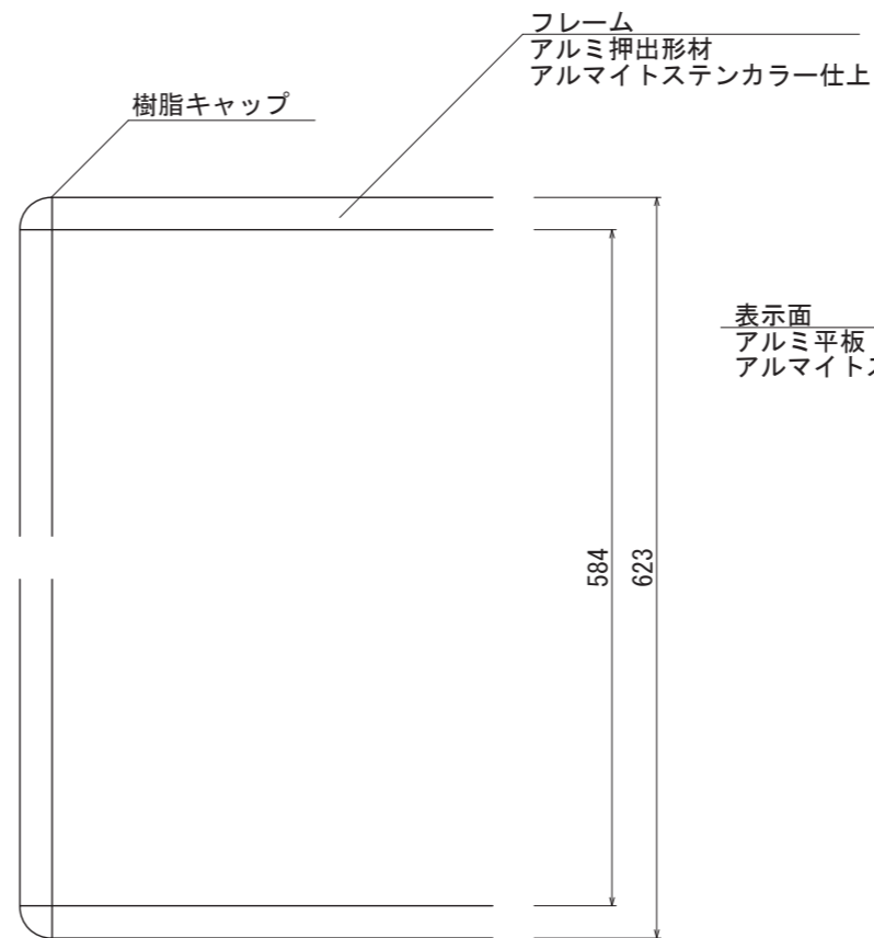
【正面図 S=1:5】
