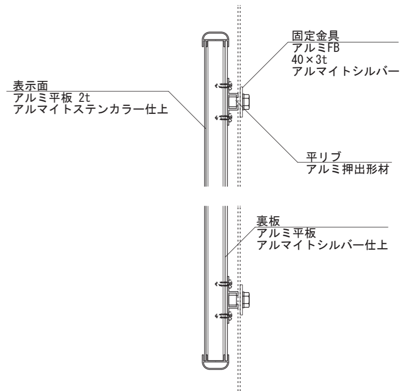
【側面図 S=1:5】
