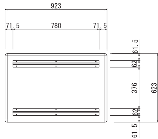
【背面図 S=1:20】
