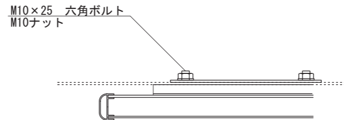
【平面図 S=1:5】
