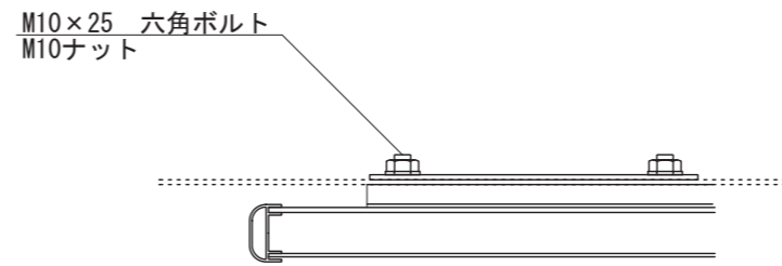
【平面図 S=1:5】
