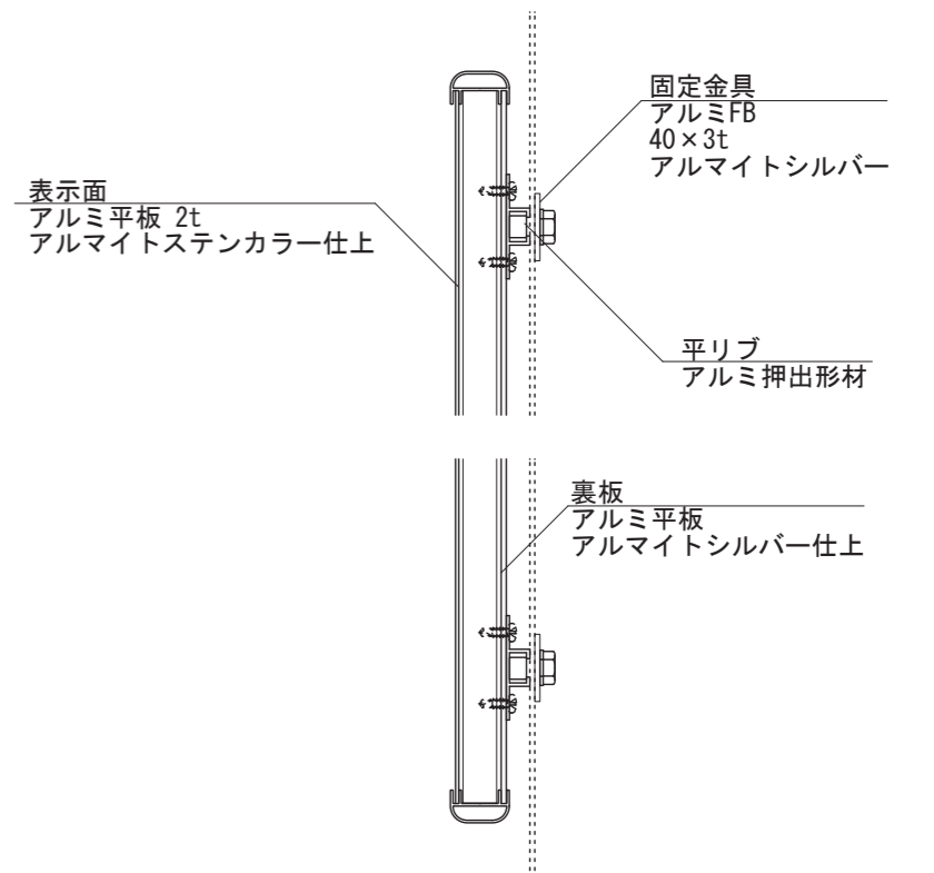
【側面図 S=1:5】
