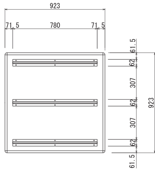
【背面図 S=1:20】
