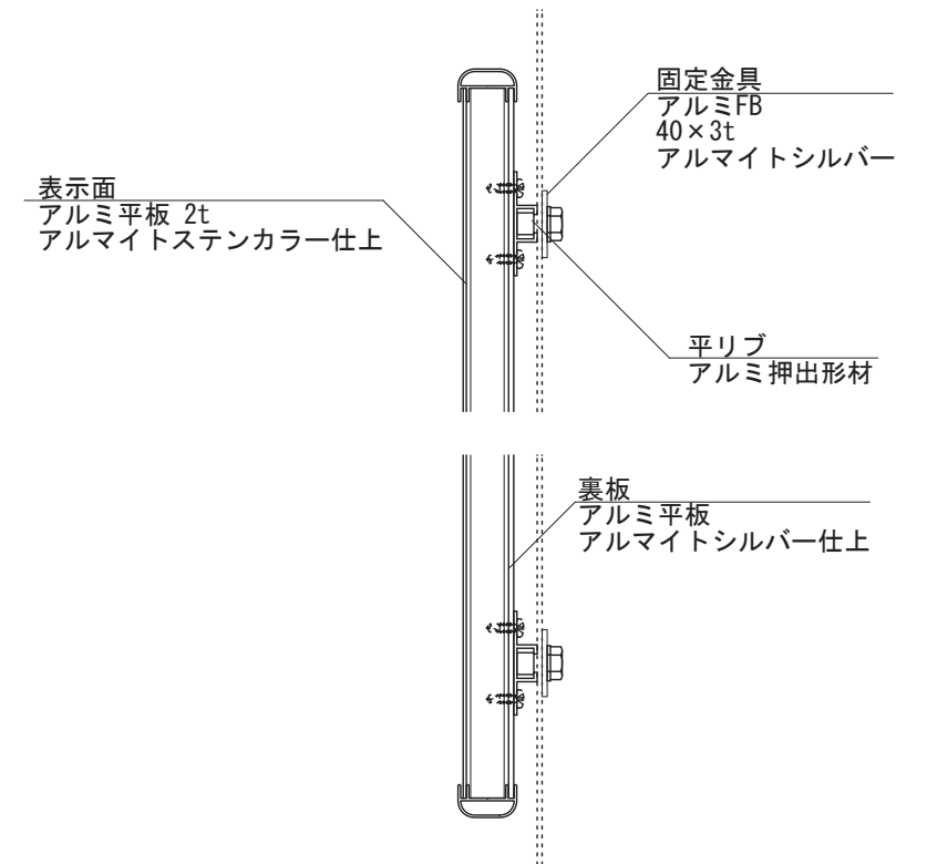
【側面図 S=1:5】
