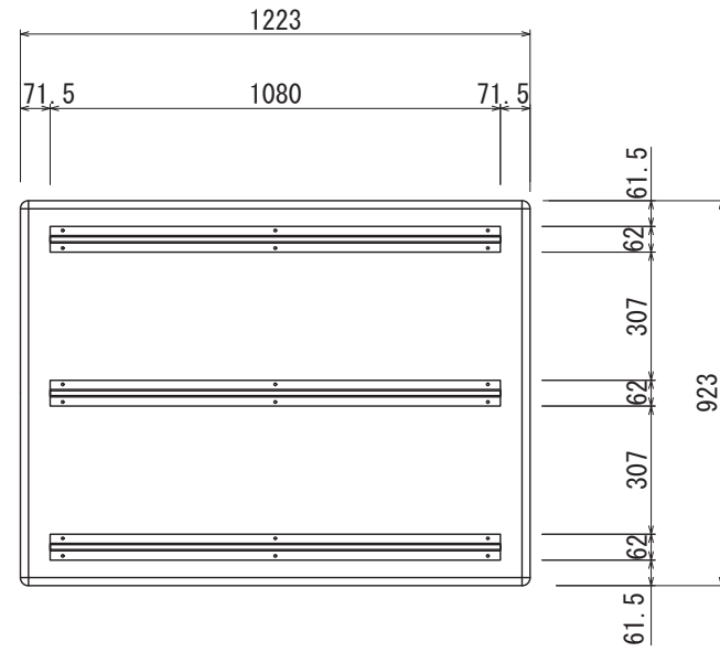
【背面図 S=1:20】
