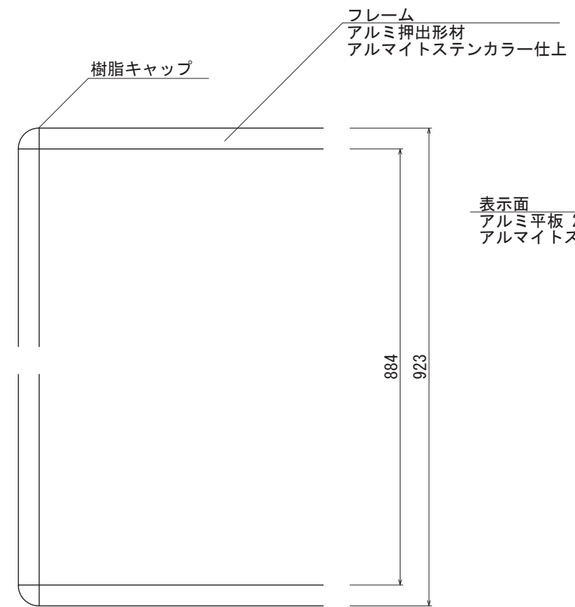
【平面図 S=1:5】
