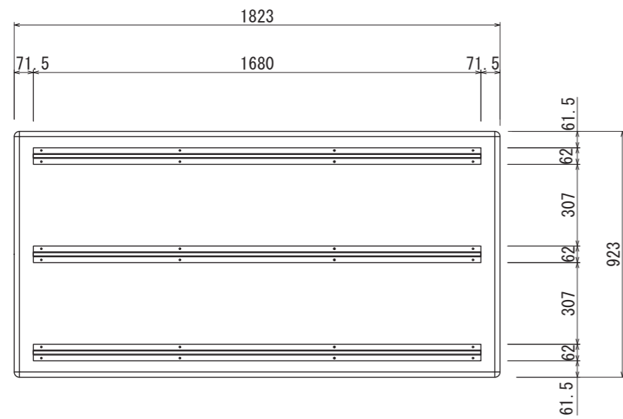
【背面図 S=1:20】
