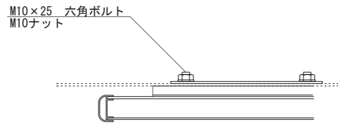
【平面図 S=1:5】
