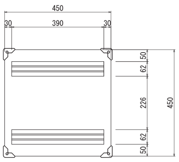
【背面図 S=1:10】
