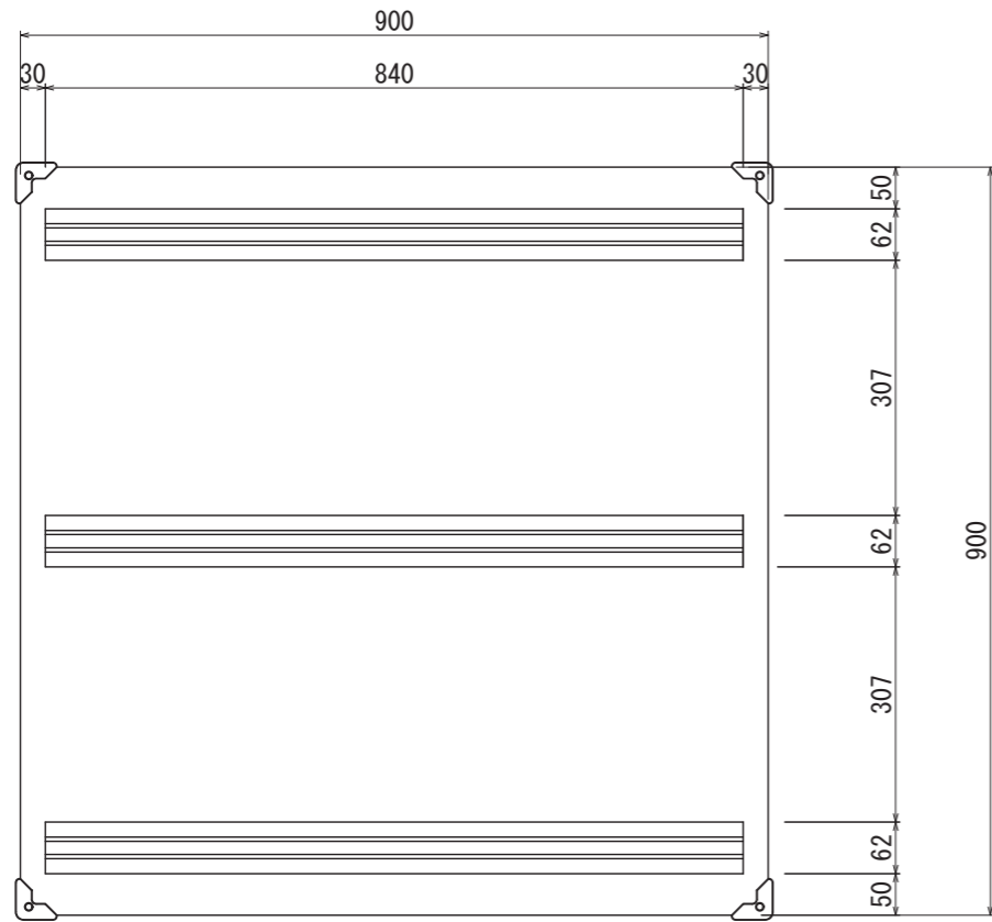
【背面図 S=1:10】
