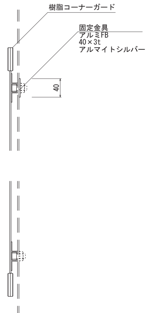
【側面図 S=1:5】
