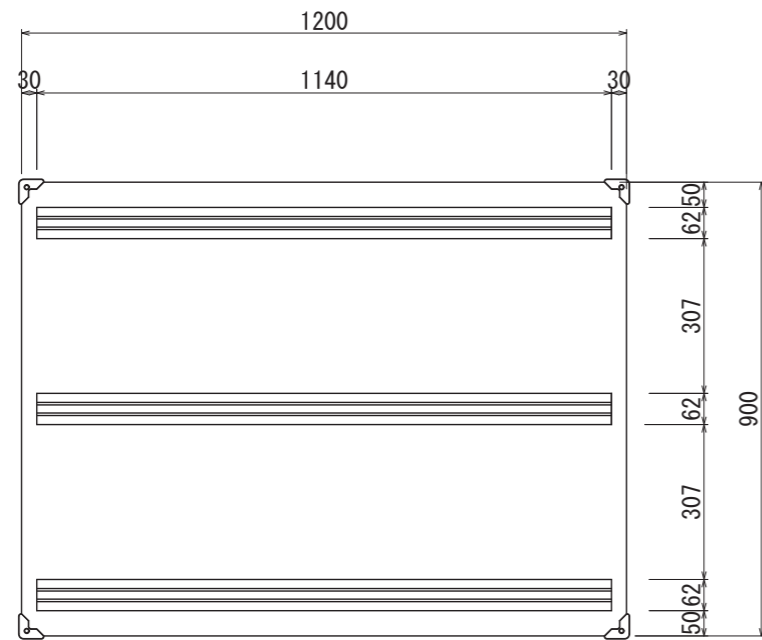
【背面図 S=1:15】
