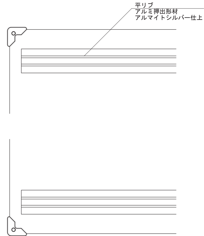
【背面図 S=1:5】
