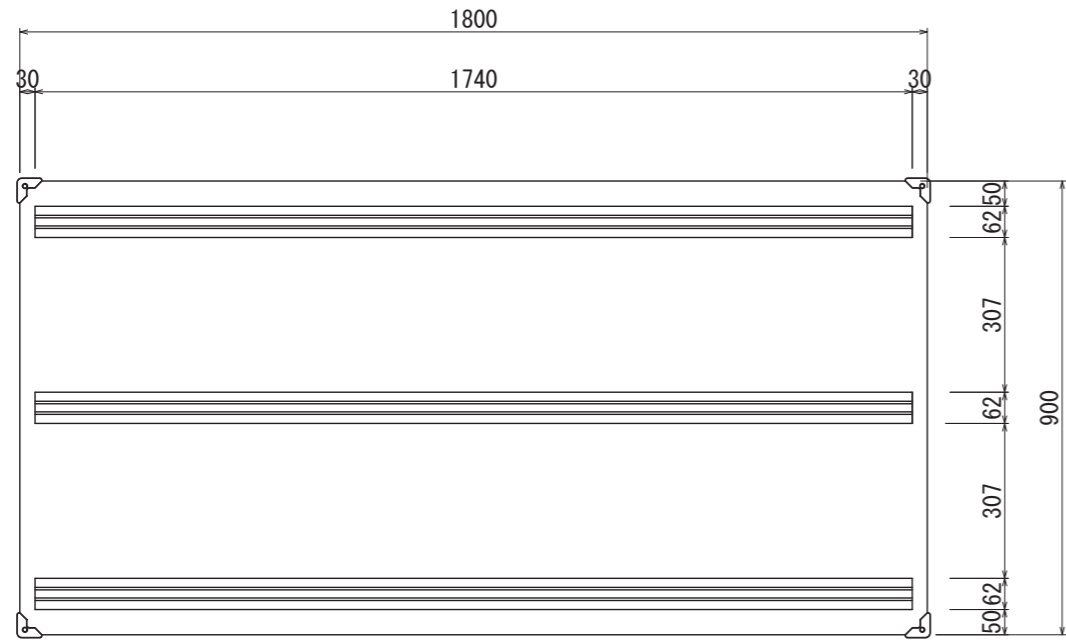
【背面図 S=1:15】
