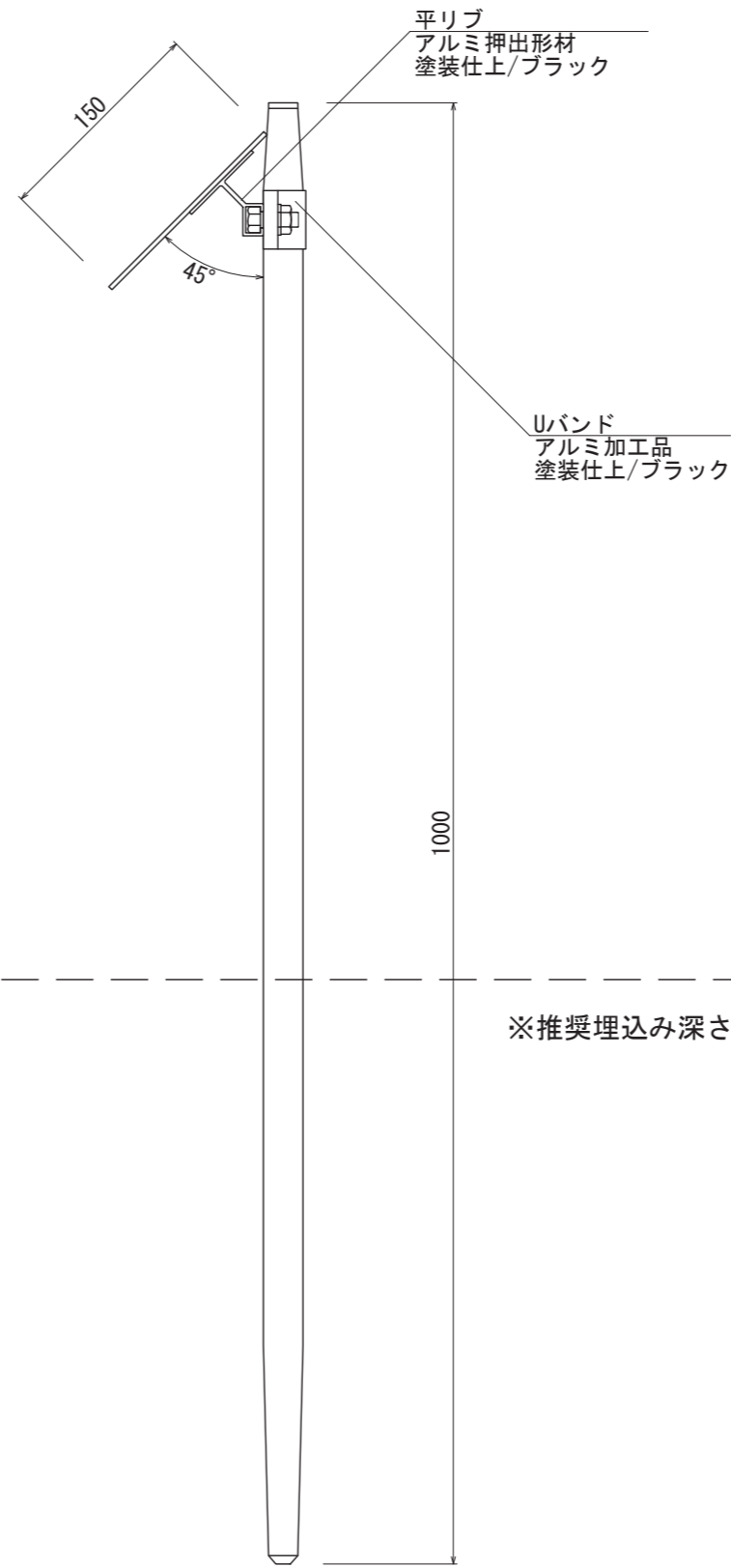
【側面図 S=1:5】
