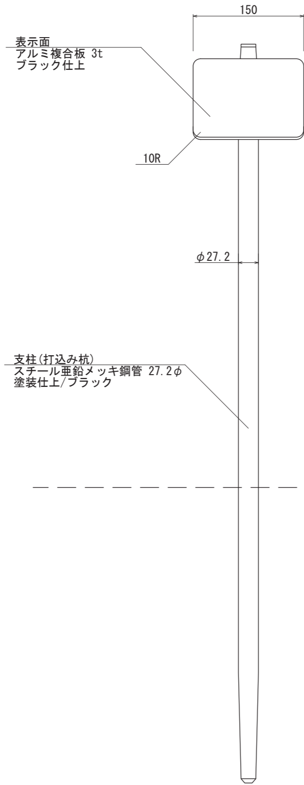
【正面図 S=1:5】
