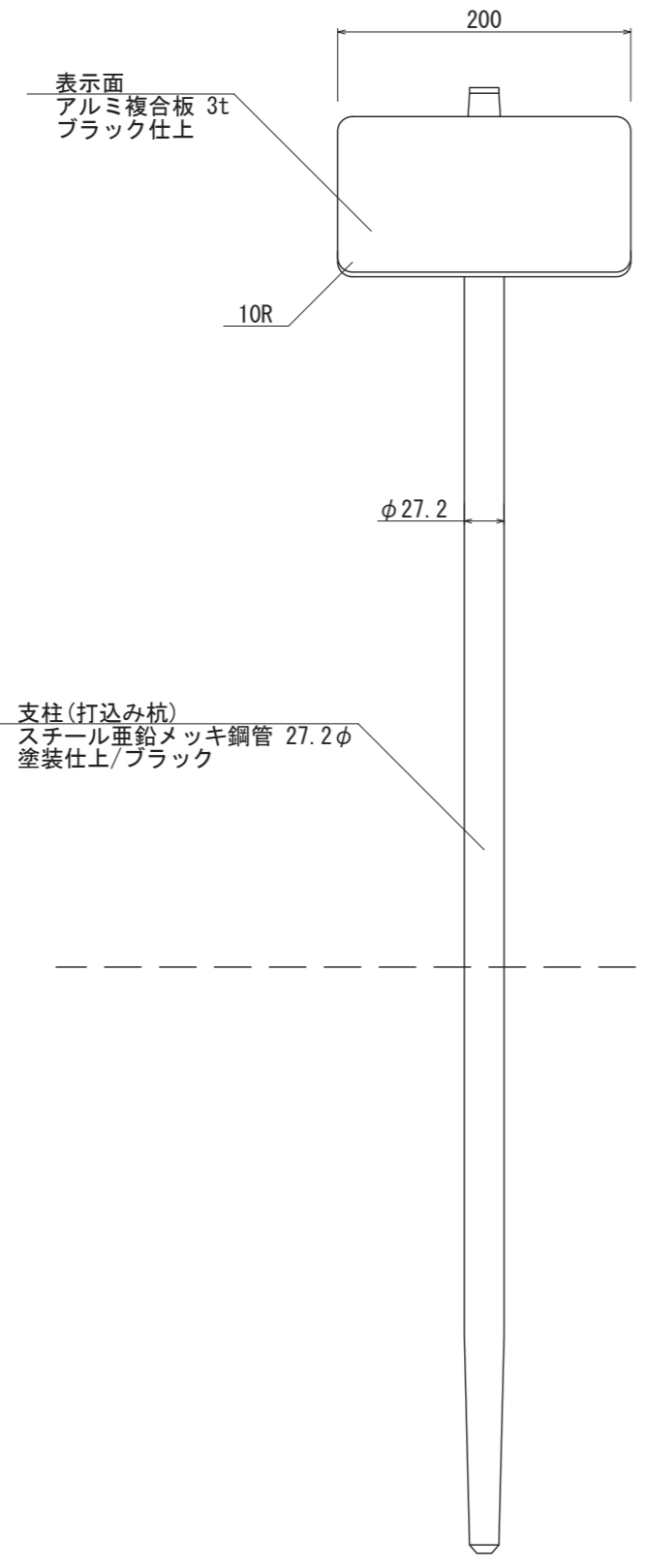
【正面図 S=1:5】
