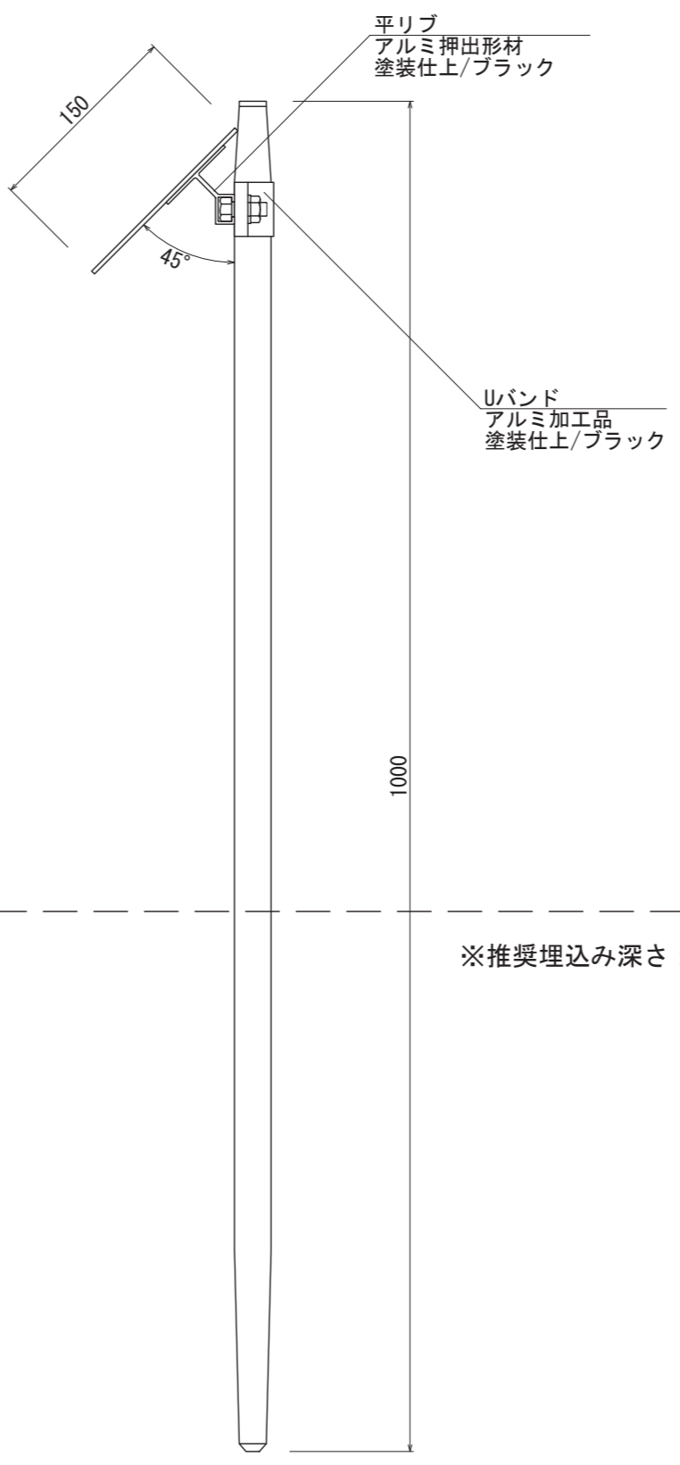
【側面図 S=1:5】
