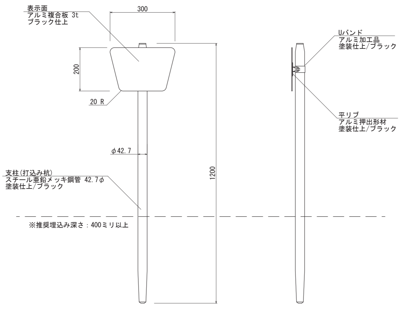
【正面図 S=1:10】
