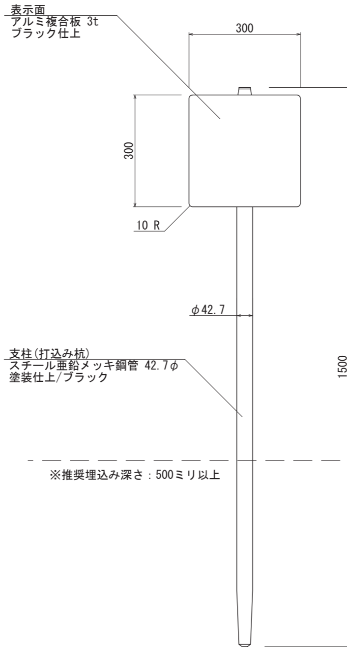
【正面図 S=1:10】
