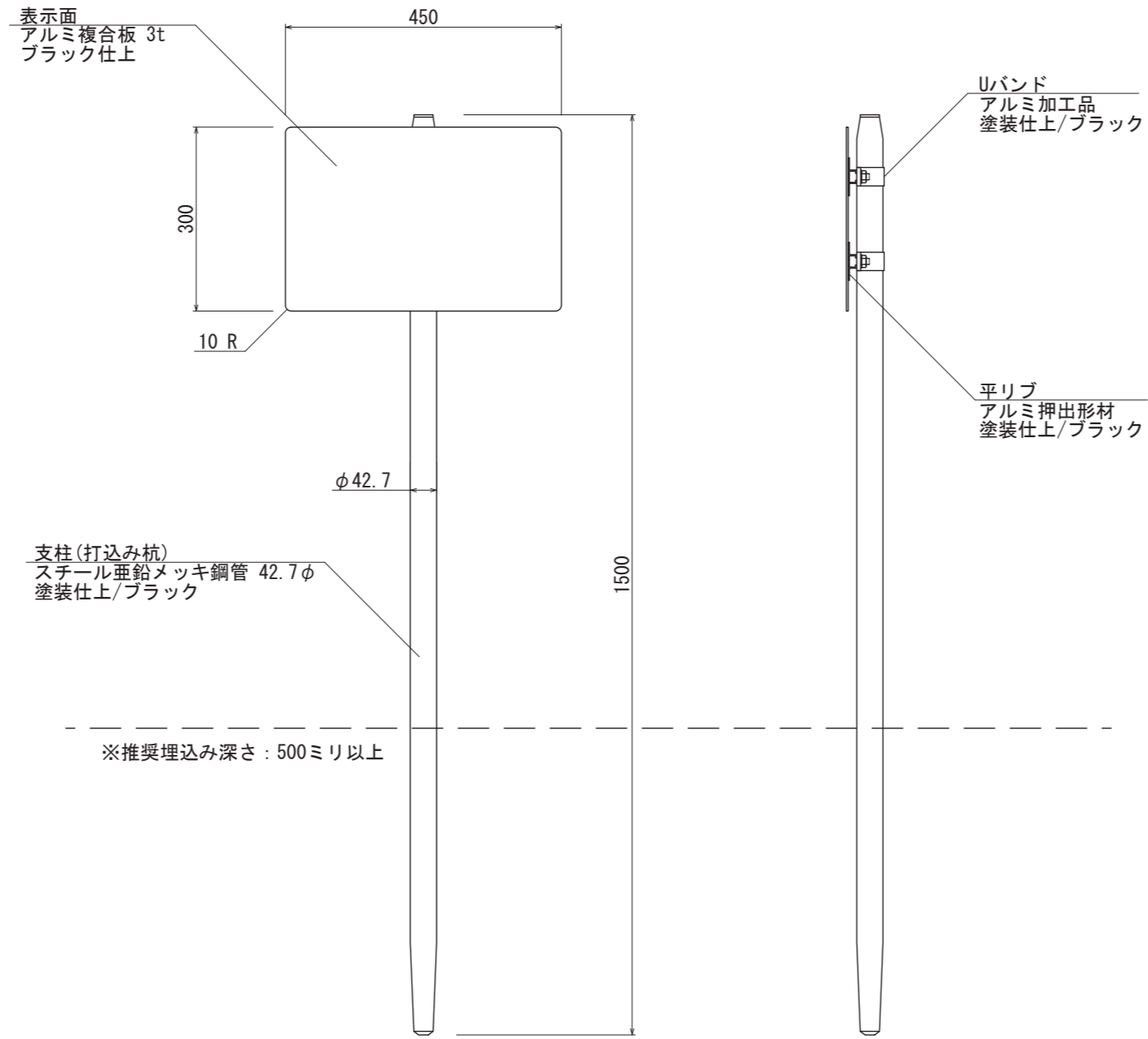
【正面図 S=1:10】
