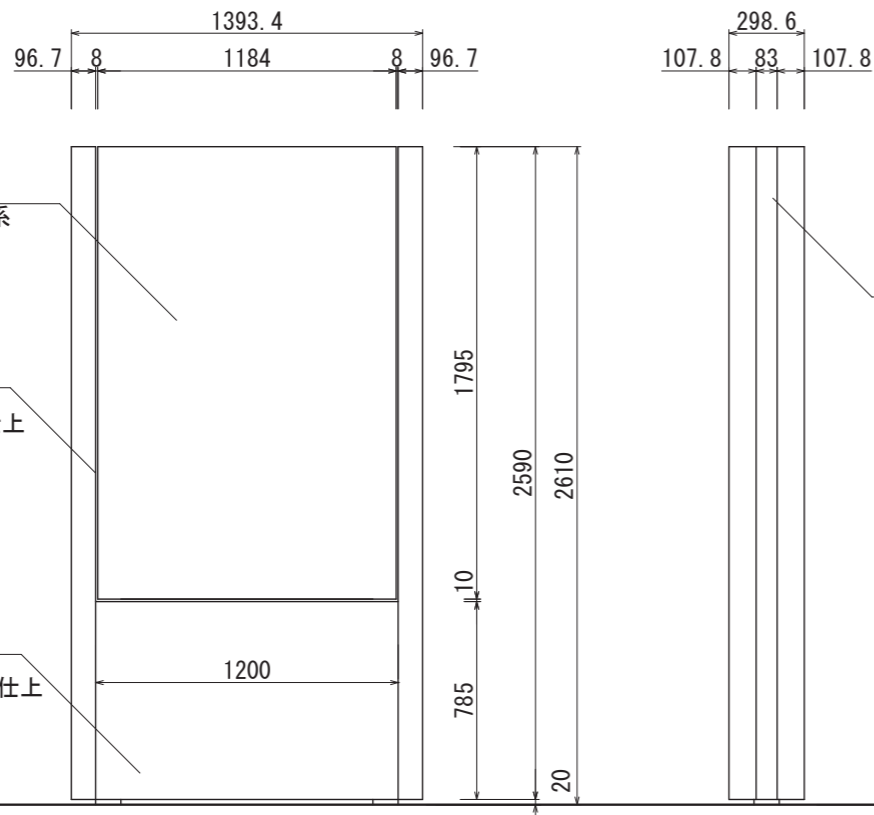
【正面図 S=1:30】
