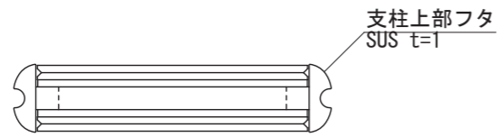
【平面図 S=1:30】
