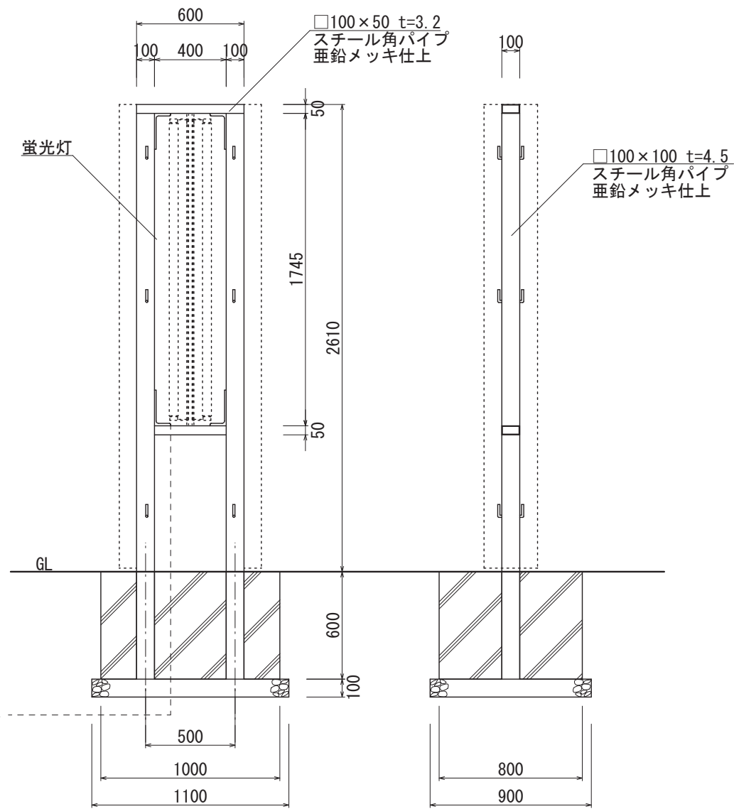
【鉄骨正面図 S=1:30】
