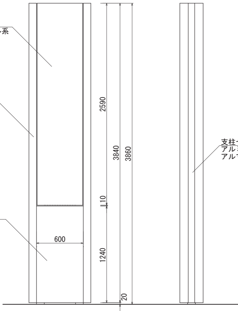
【正面図 S=1:30】
