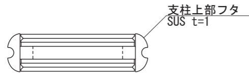
【平面図 S=1:30】
