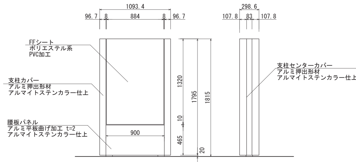
【正面図 S=1:30】
