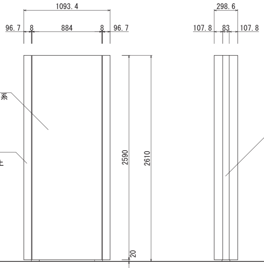
【正面図 S=1:30】
