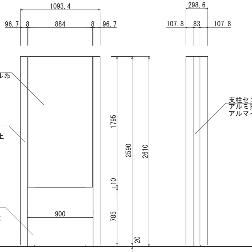
【正面図 S=1:30】
