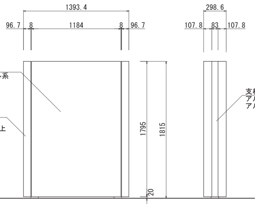
【正面図 S=1:30】
