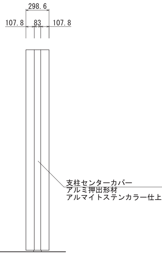
【側面図 S=1:30】
