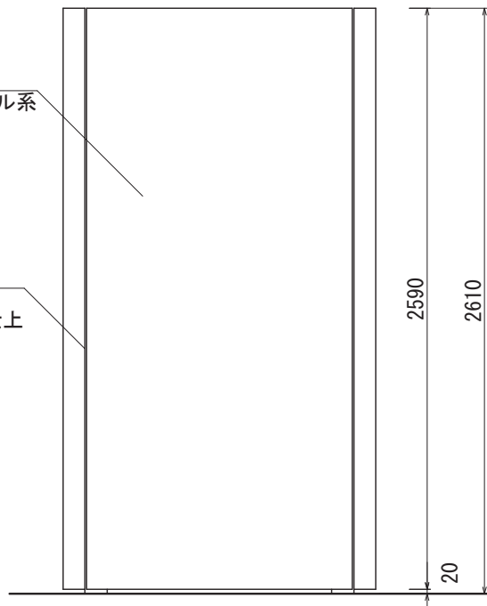
【正面図 S=1:30】
