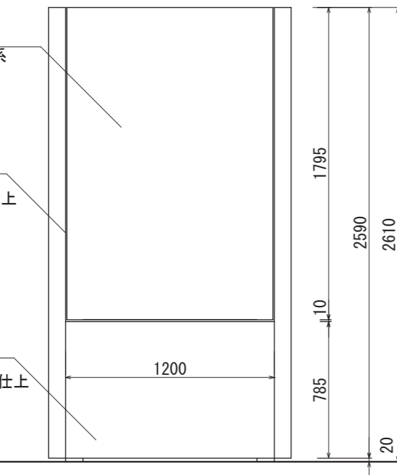
【正面図 S=1:30】
