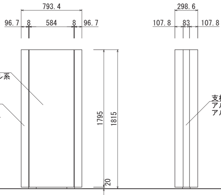
【正面図 S=1:30】
